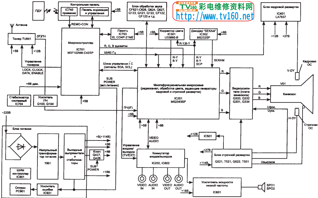
Структурная схема
