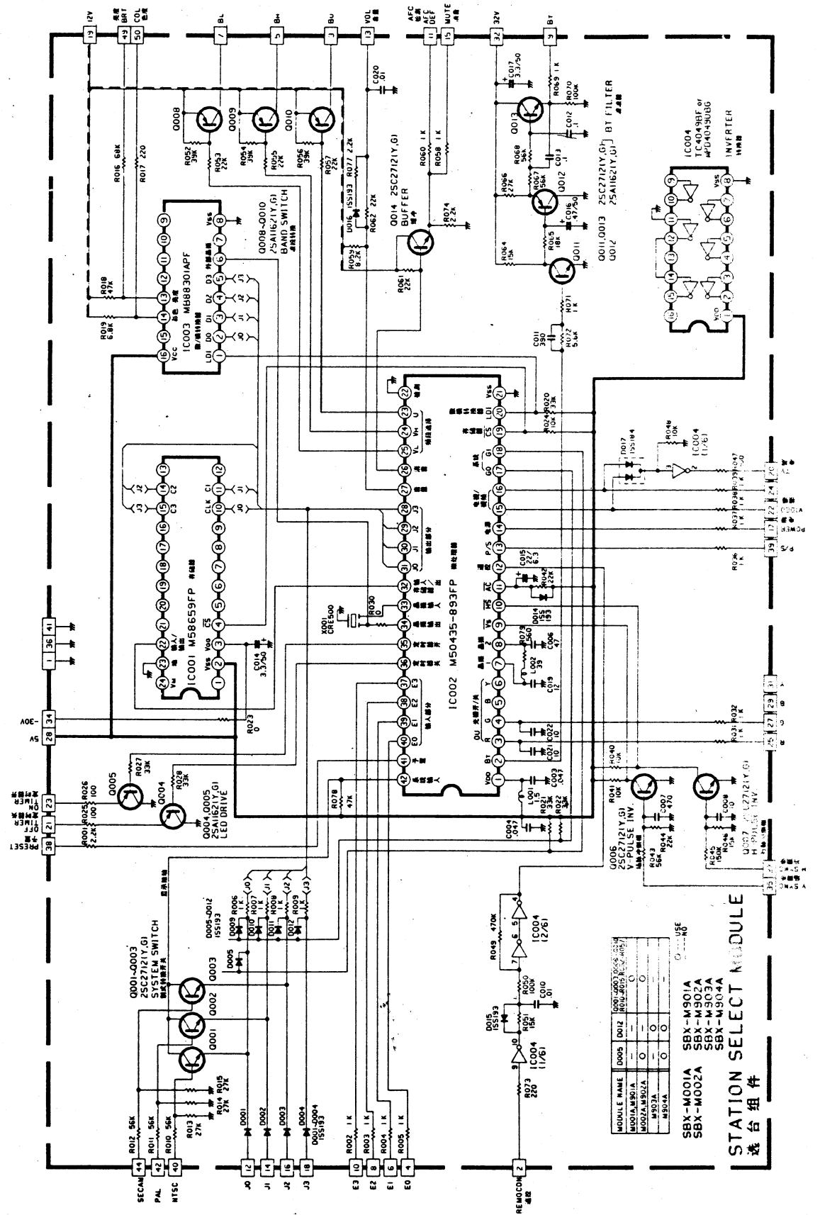
选台组件原理图 S. SELECT MODULE SCHEMATIC DIAGRAM (SBX-M002A)
