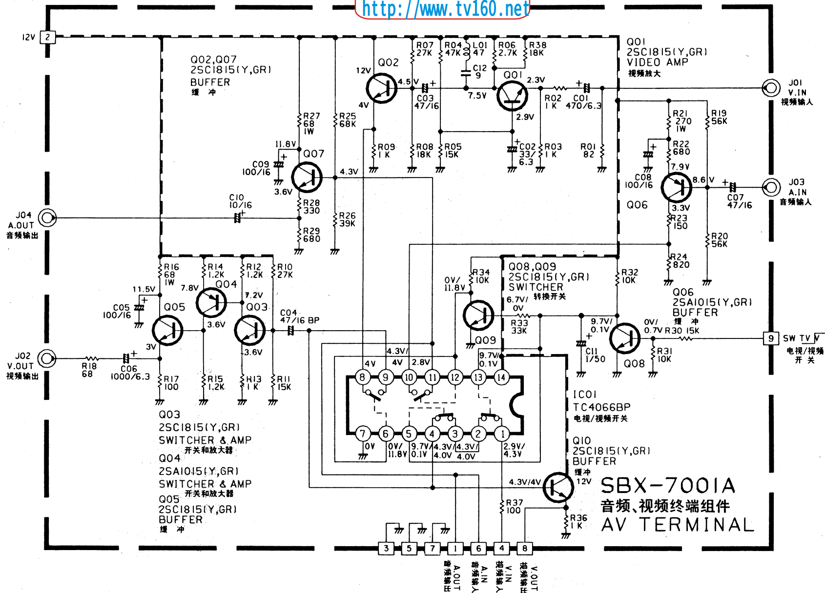
音频、视频终端组件原理图 AV TERMINAL SCHEMATIC DIAGRAM (SBX-7001A)
