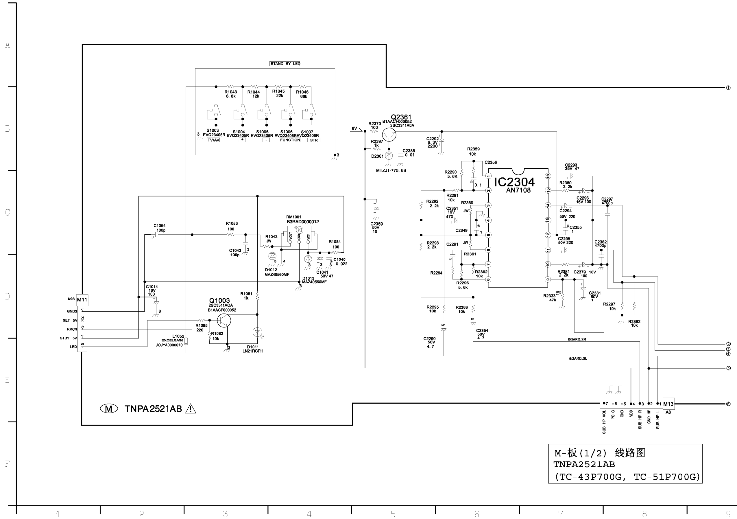
15. 13. M-板 (1/2) 线路图
