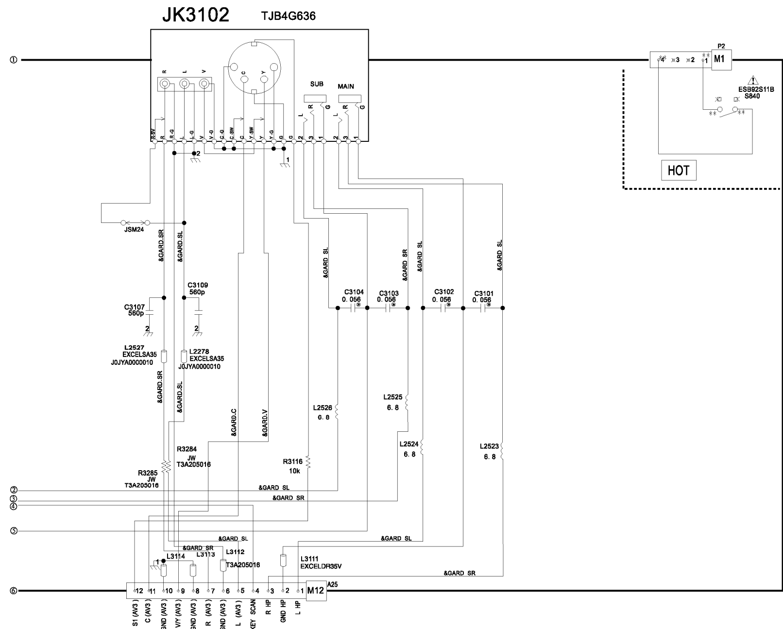
M-板 (2/2) 线路图 TNPA2521AB (TC-43P700G, TC-51P700G)
