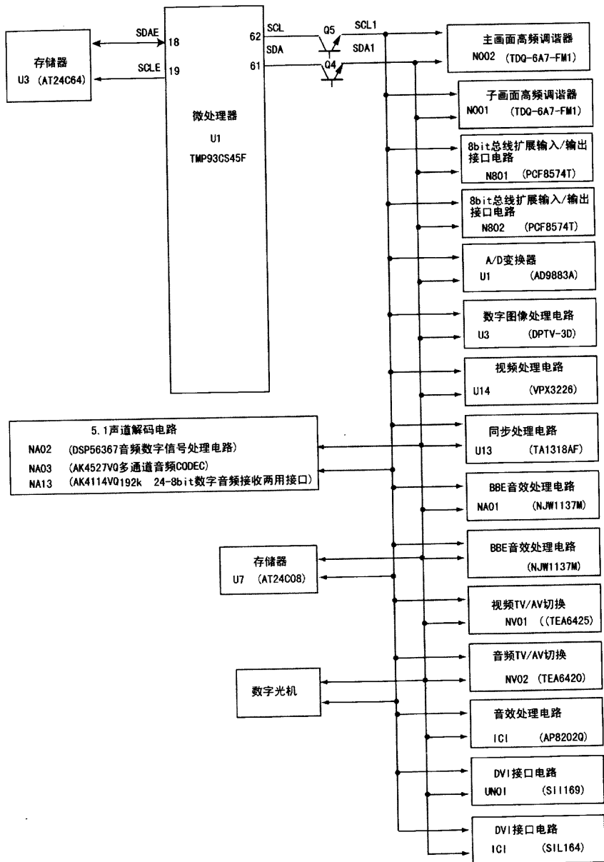
图 23-1 长虹 DLP 背投影电 I²C 总线控制连接方框图
