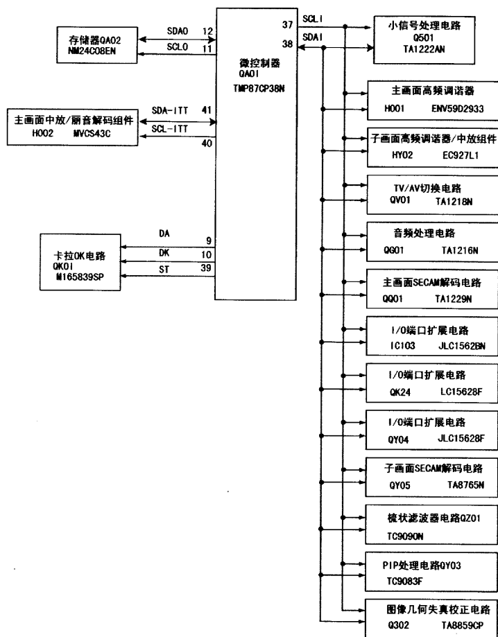
图 3-1、NC-6 机心 PC 总线控制连接方框图
