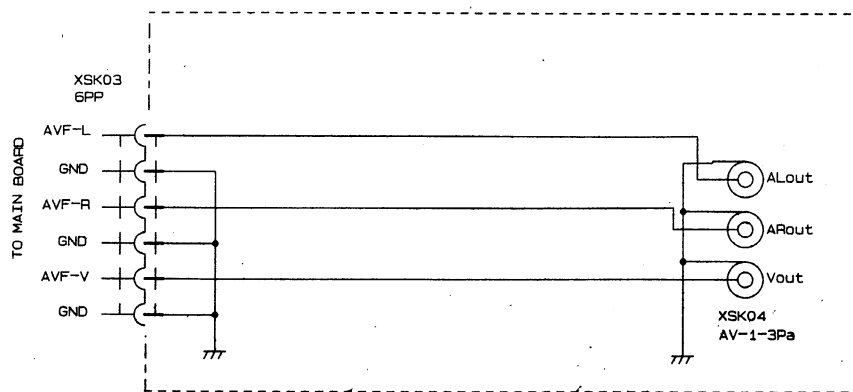
L AV Board JUC2.025.013
