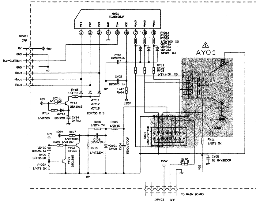
Y Board JU7. 820. 1586-3
