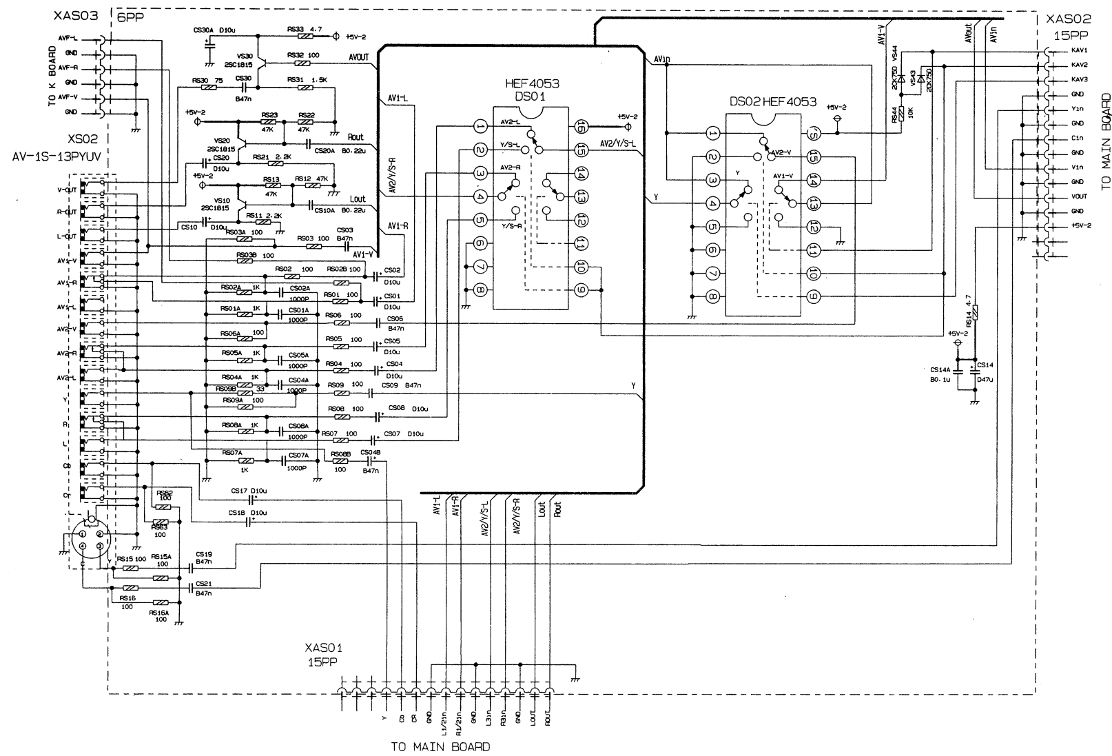
AV BOARD JUC7.820.031
