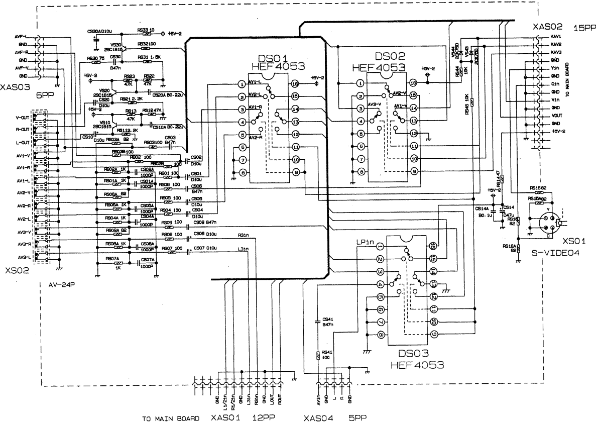
AV Board JU7.820.1585-1
