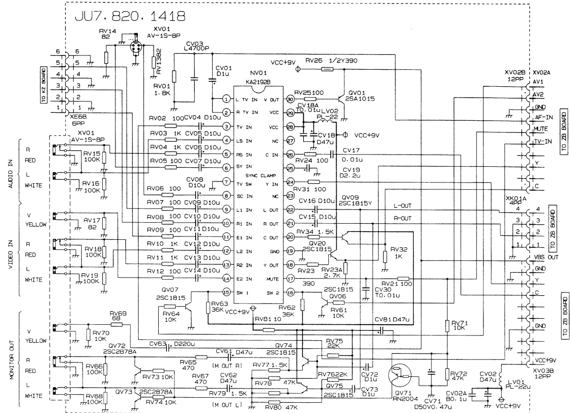
R2516N AV BOARD
