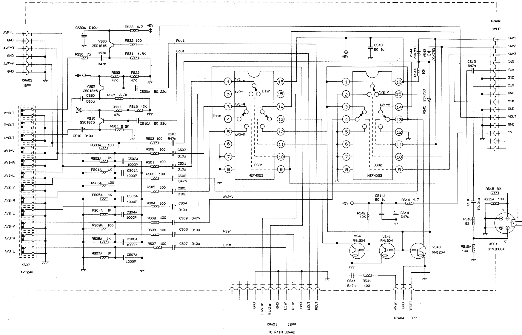
AV Board JU7.820.1585
