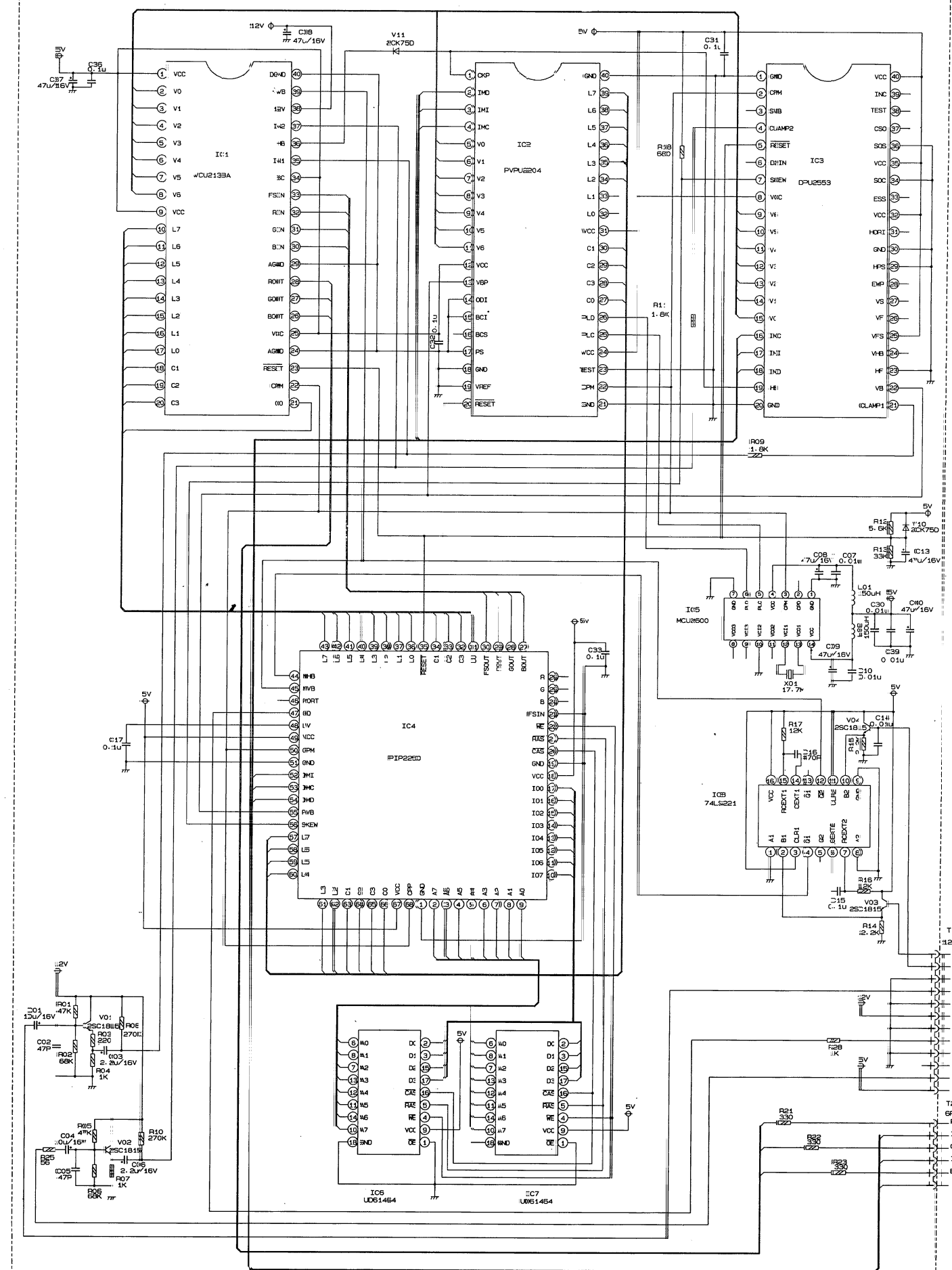
PW 板电路图
