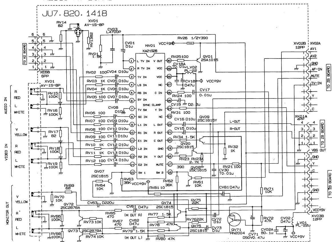
N2516 AV BOARD
