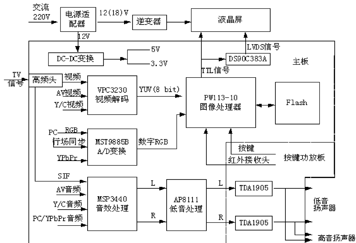
LP03机芯E系列液晶电视信号流程框图
