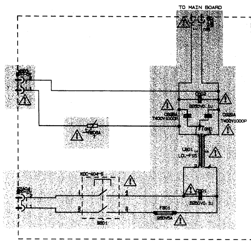
POWERBOARD JUC7.820.1036
