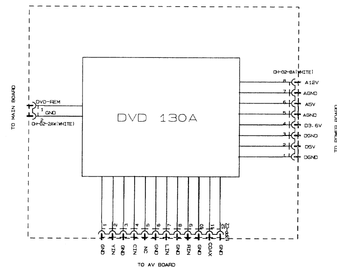
DVD 组件
