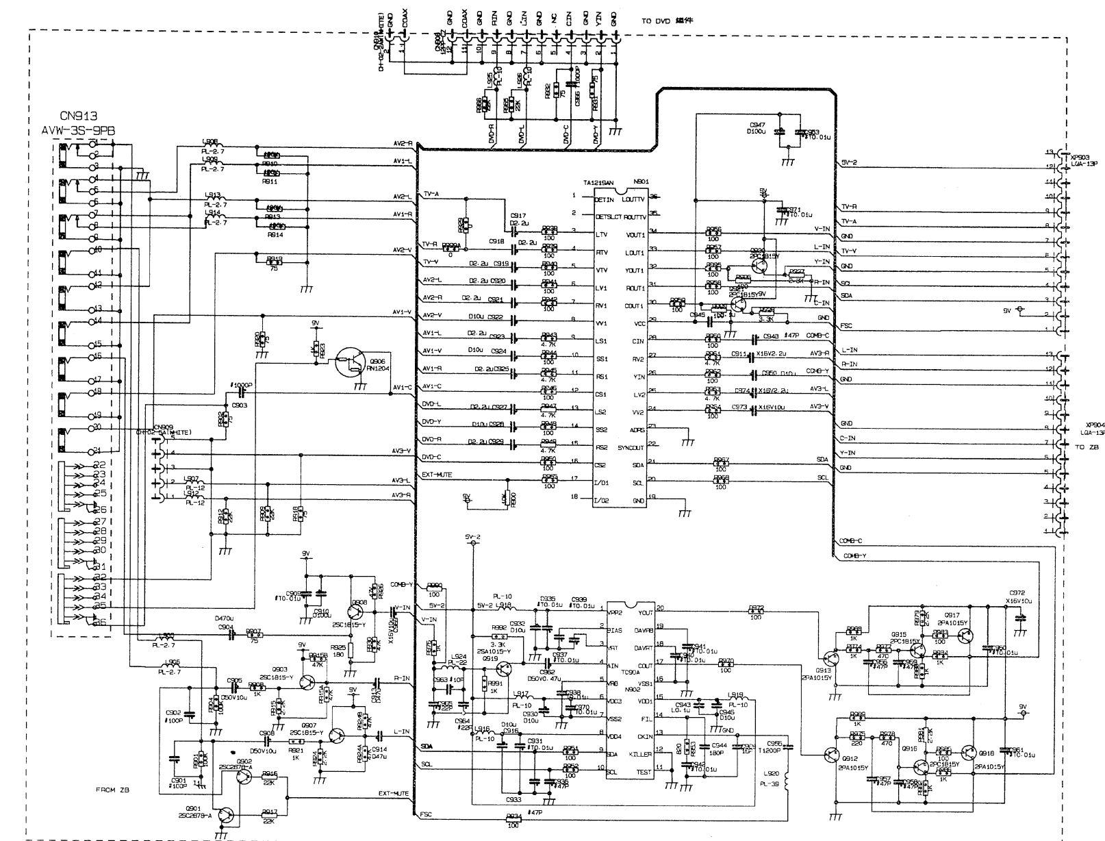
AV BOARD JUC7.820.1087
