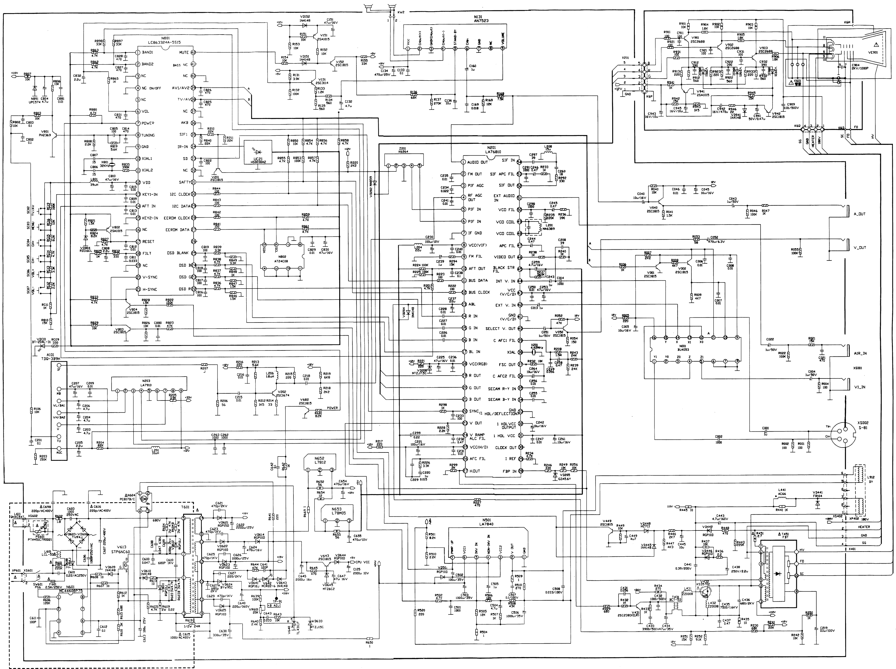
海信牌 TC2102G/TC2175G 彩色电视机原理图
