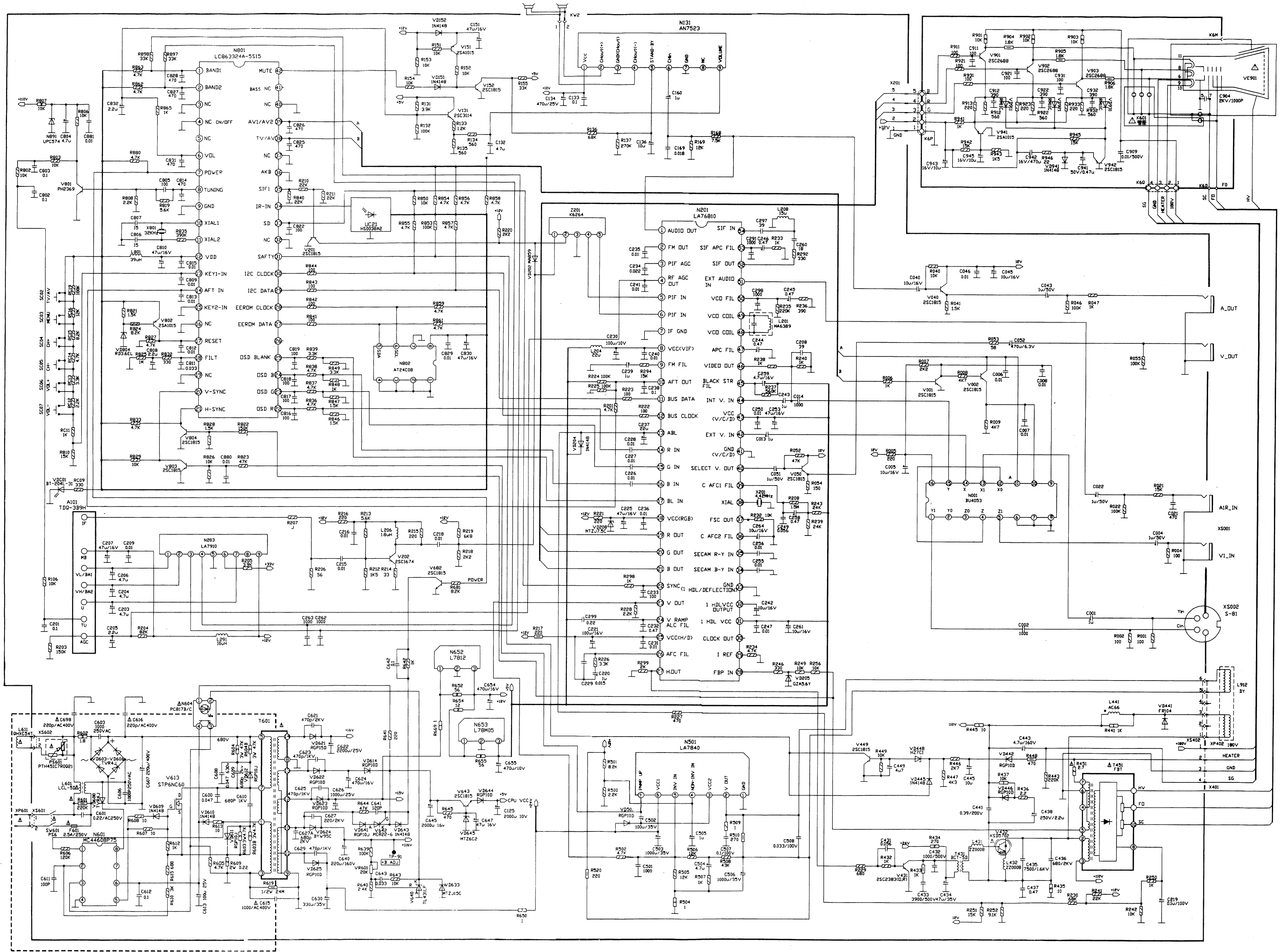
海信牌 TC2102GD/TC2175GD 彩色电视机原理图
