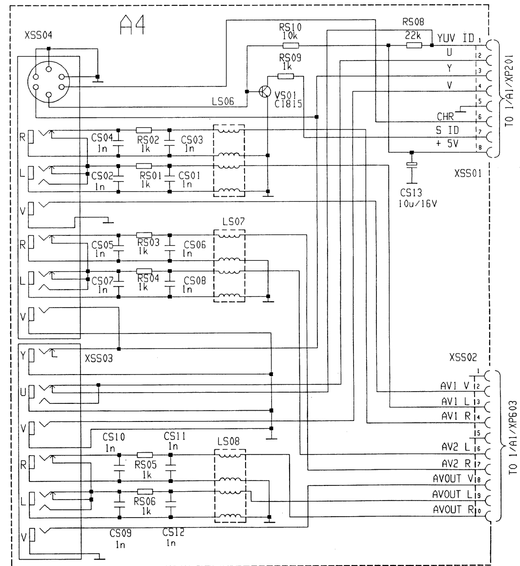
海信牌 TC2911G 型彩色电视机电路图 (A2、A3、A4、A6、A7、A8板) 第2页
