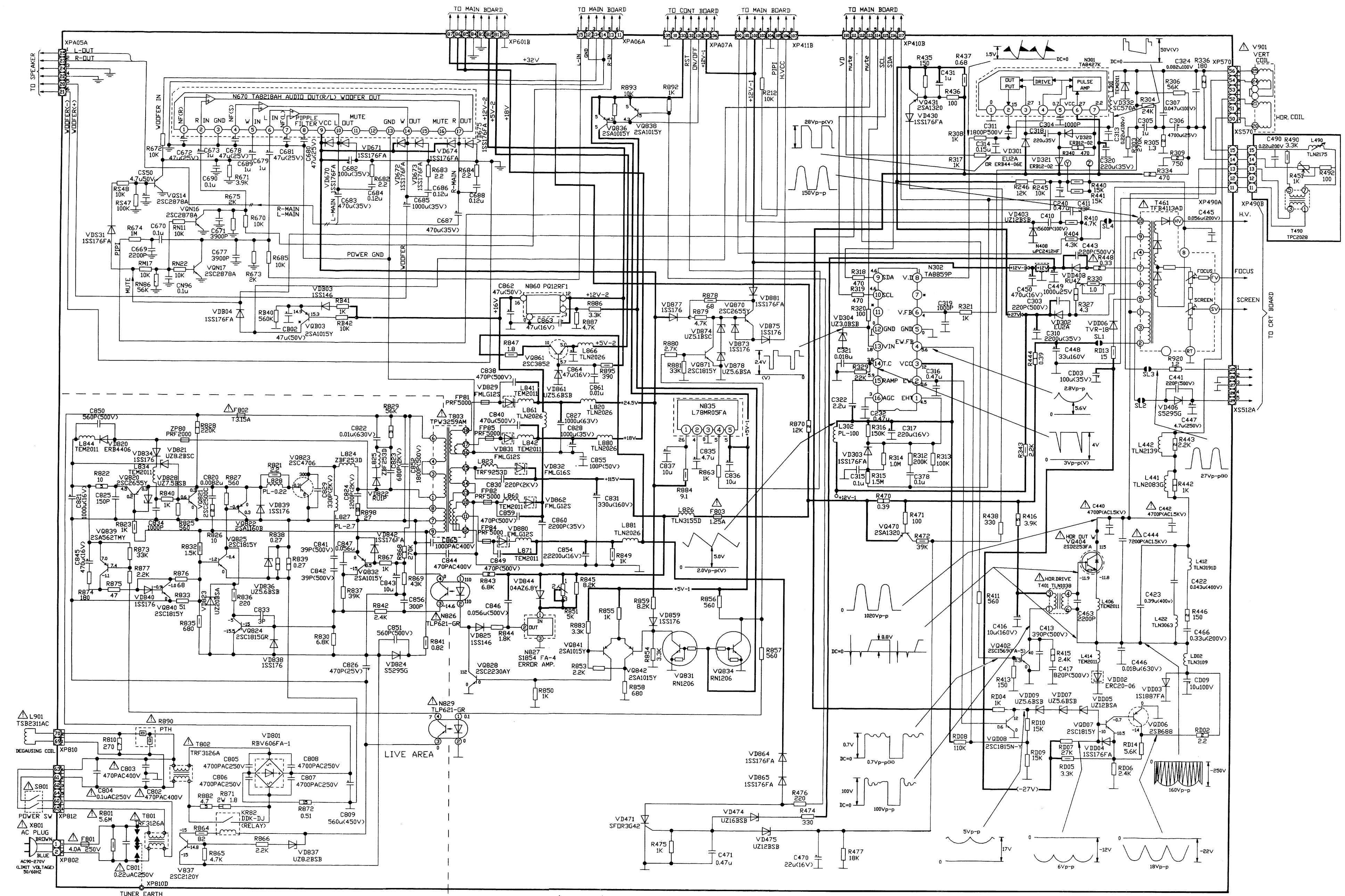
电源、偏转、音频功放部分线路 海信牌彩色电视机电路图（TC2939 系列）2/4
