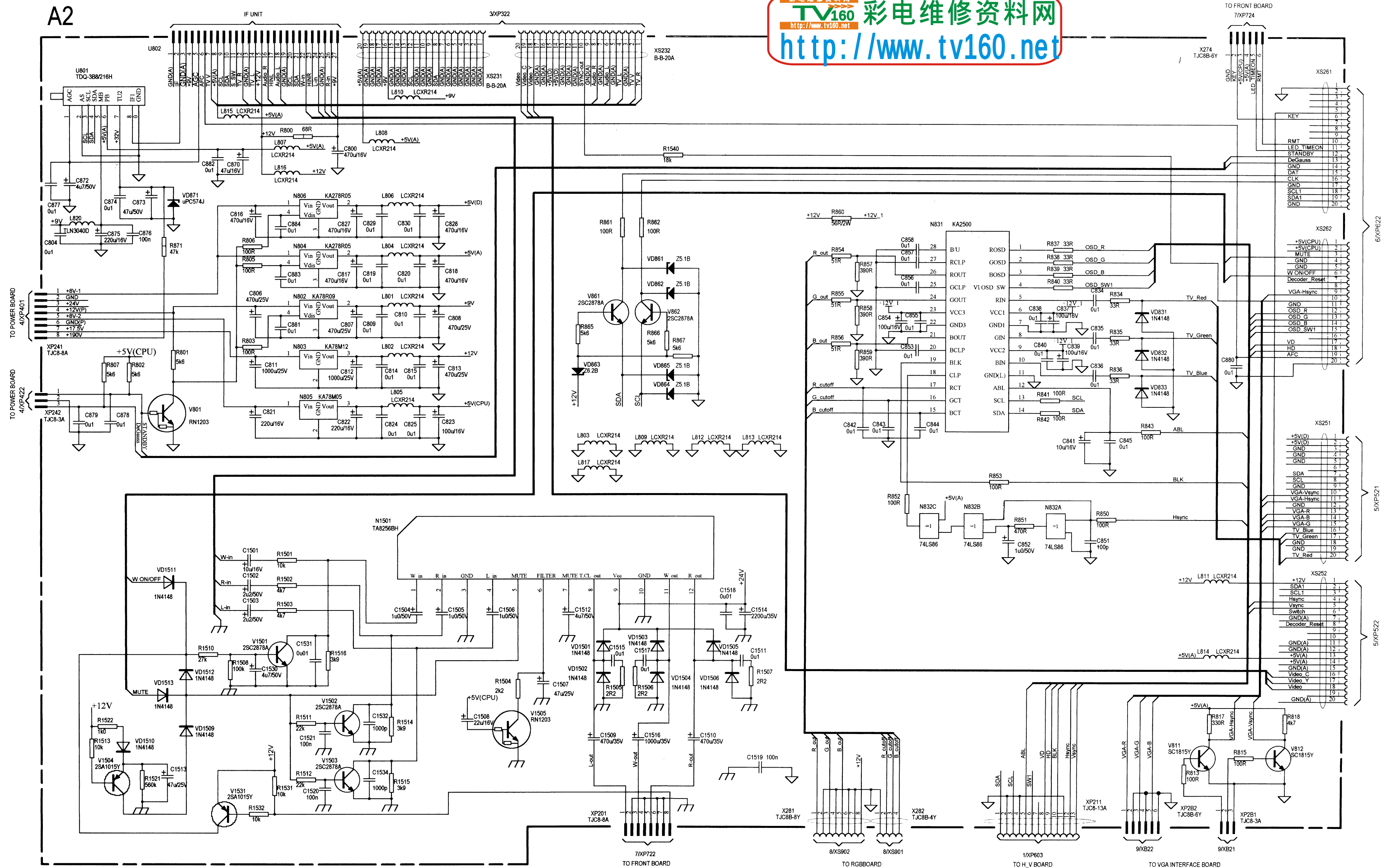
海信牌 DP2988H 型彩色电视机电路图 (A2 板) 共 6 页 第 2 页
