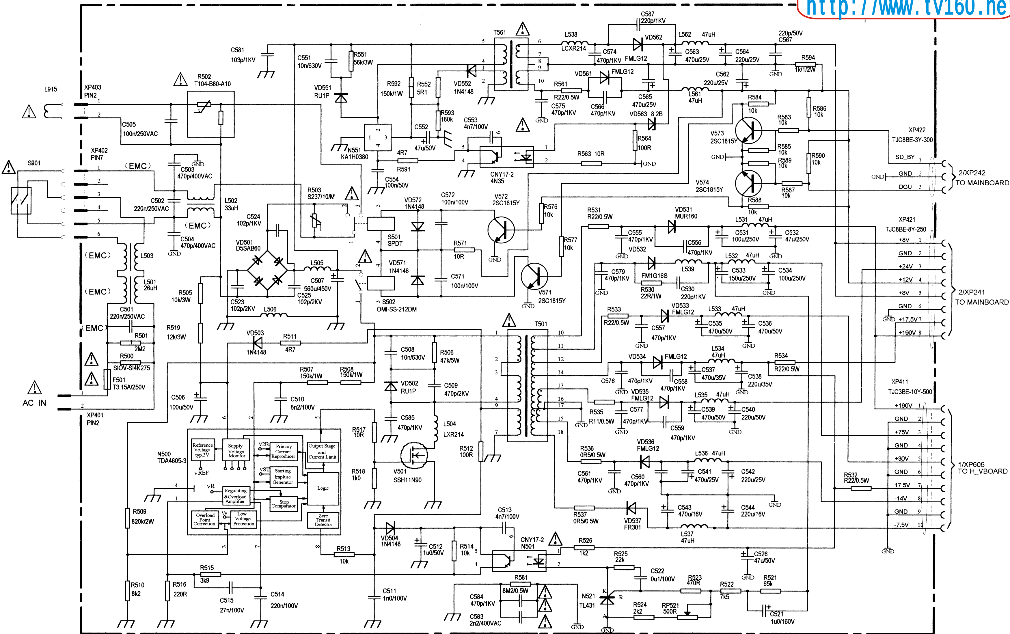
海信牌 DP2988H 型彩色电视机电路图 (A4 板) 共 6 页 第 5 页
