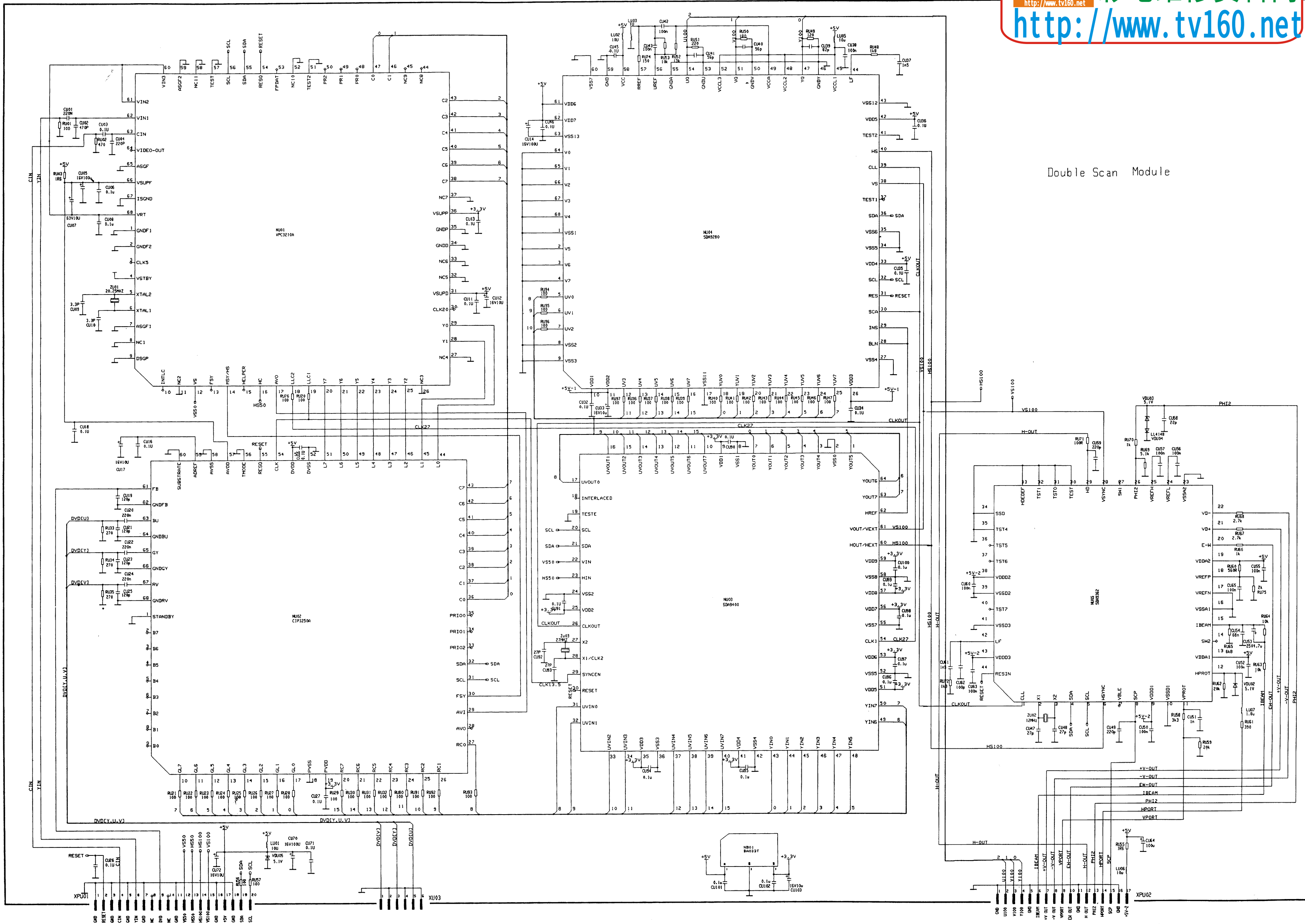
海信牌 eTV-2988 型网络电视机电路图 (A4板) 第4页
