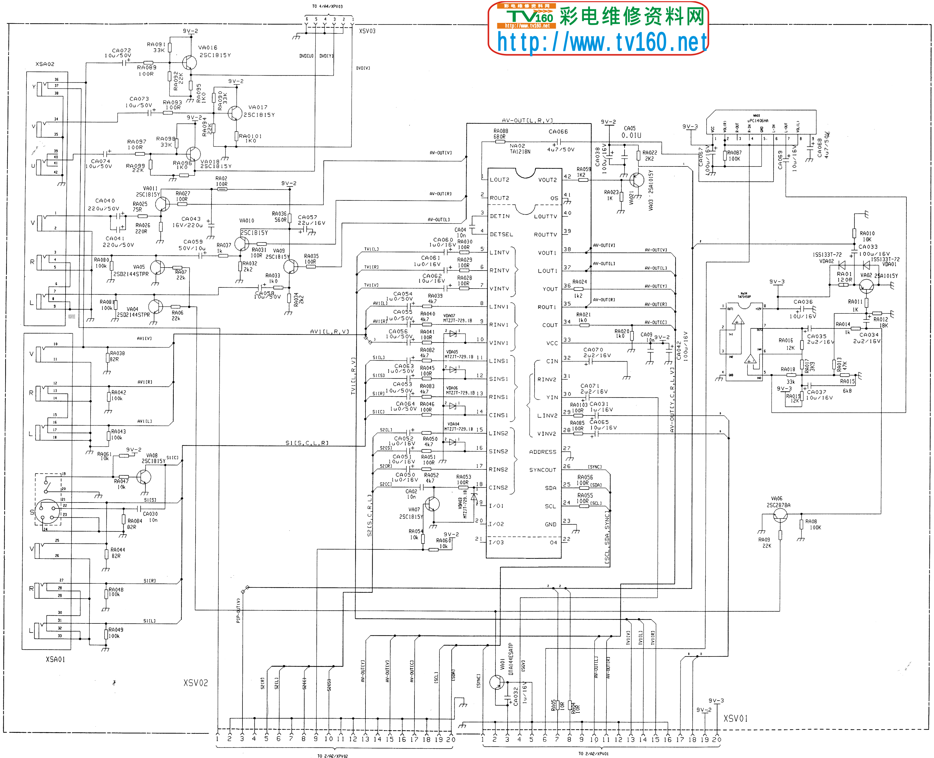
海信牌 eTV-2988 型网络电视机电路图 (A6板) 第6页
