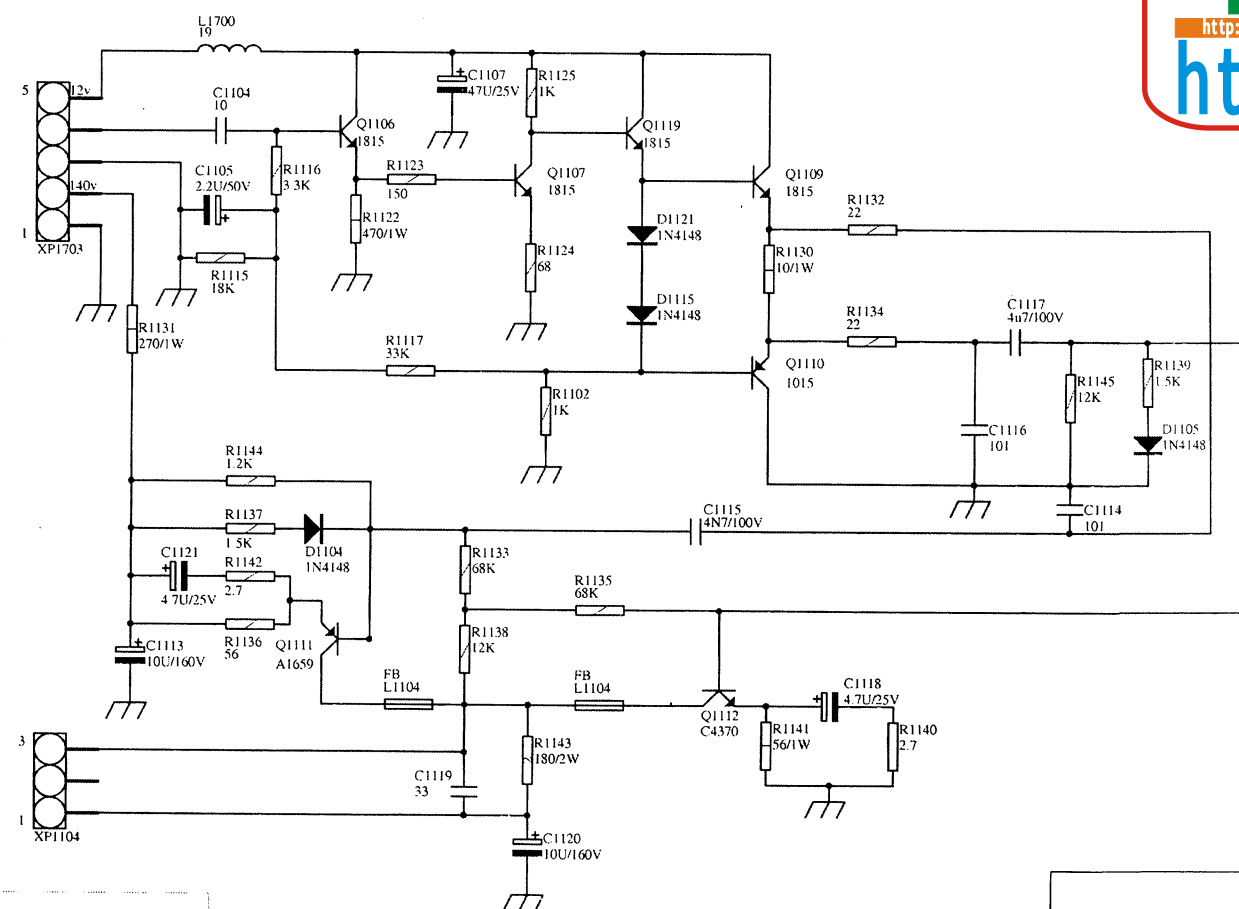
调速板 A5
