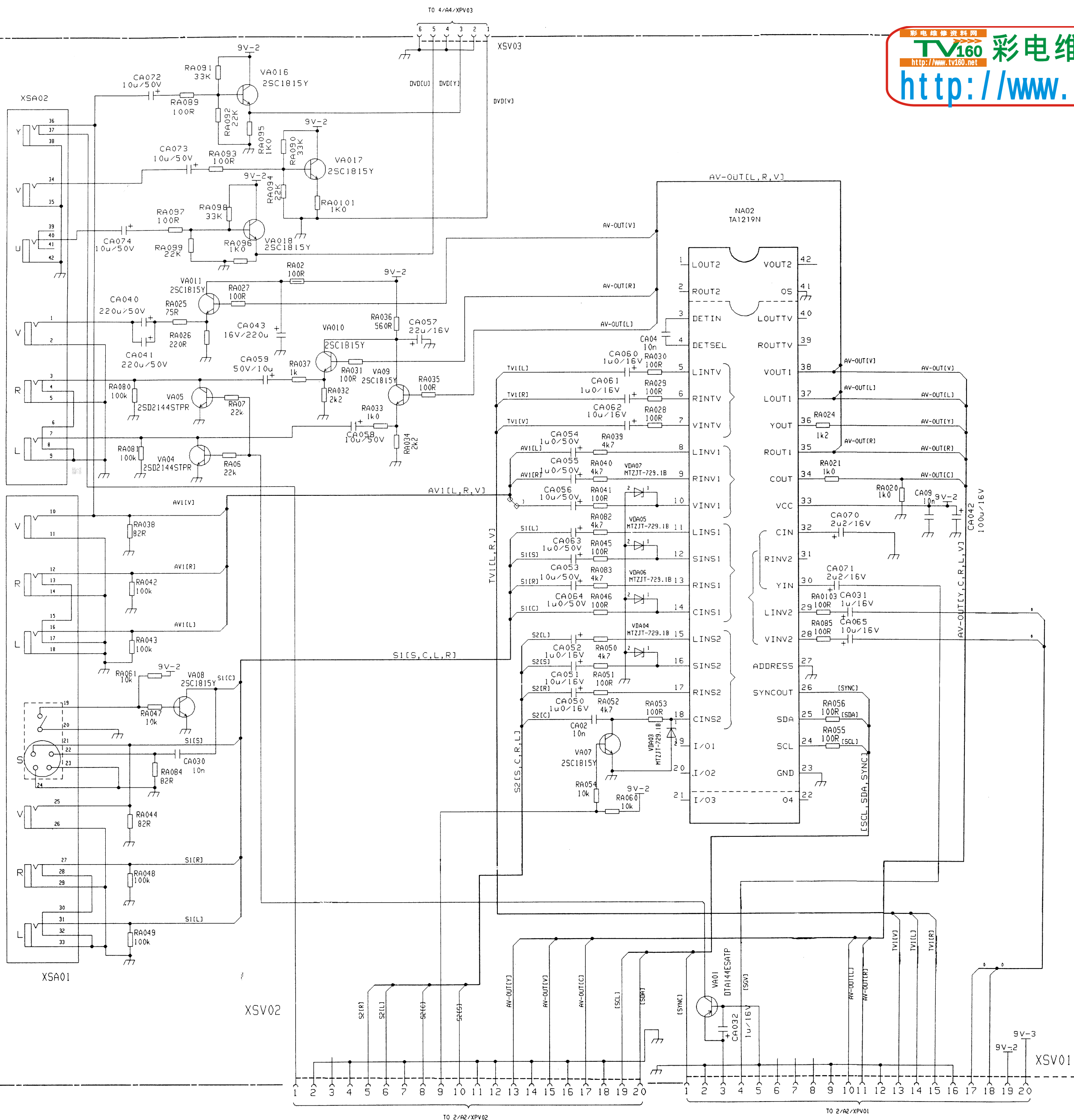
海信牌 TDF2900型彩色电视机电路图 (A6板) 共6页 第6页
