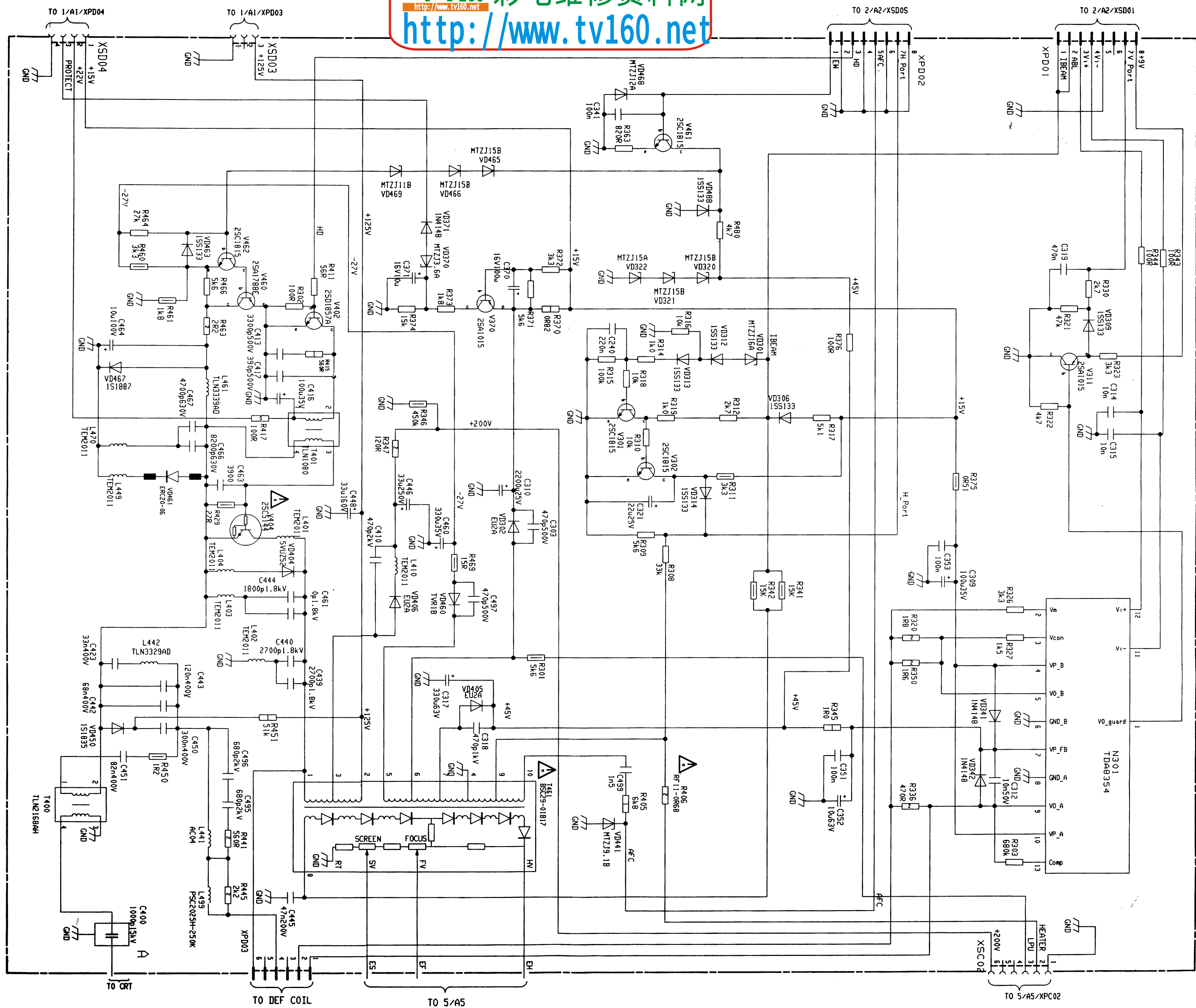
海信牌TDF2988型彩色电视机电路图 (A3板) 第3页
