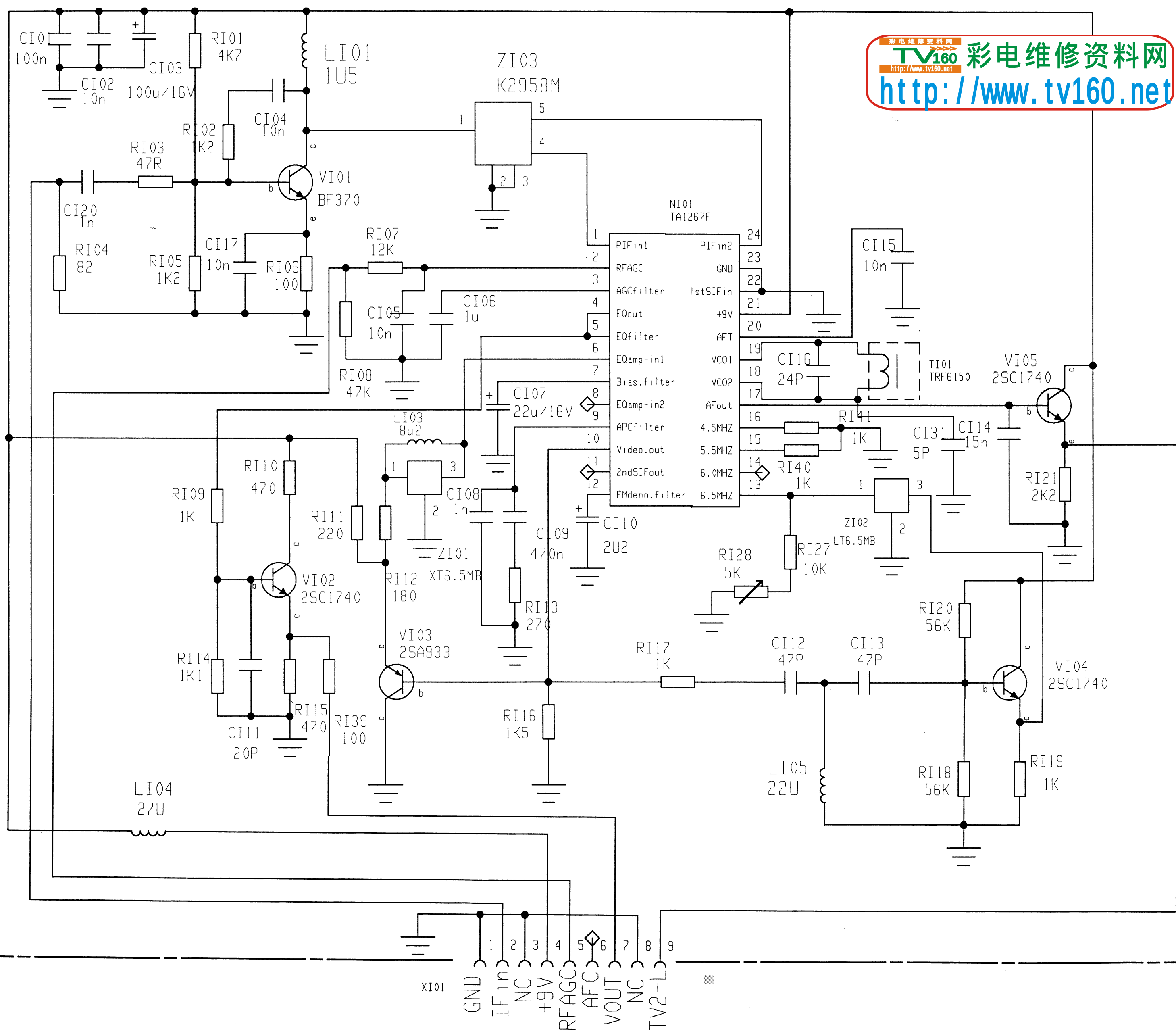
海信牌TDF2988型彩色电视机电路图（A9板）第7页
