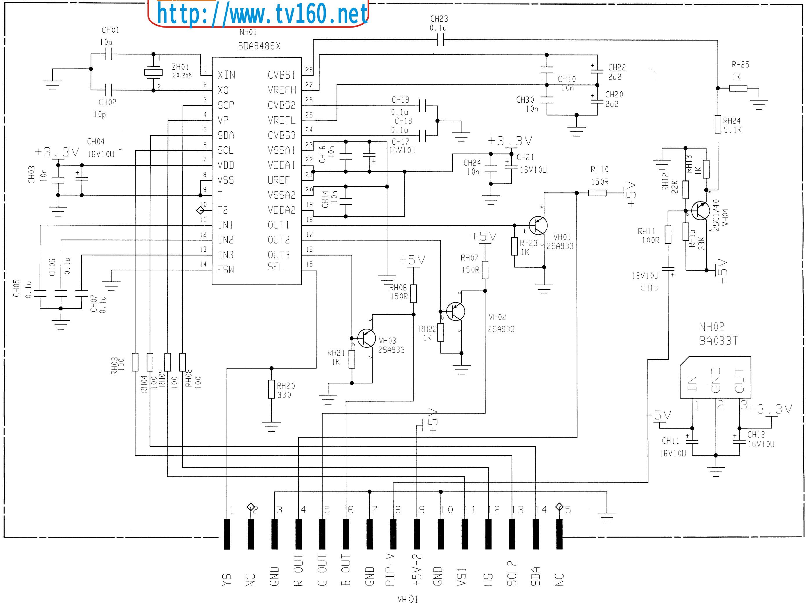
海信牌TDF2988型彩色电视机电路图（A10板）第8页
