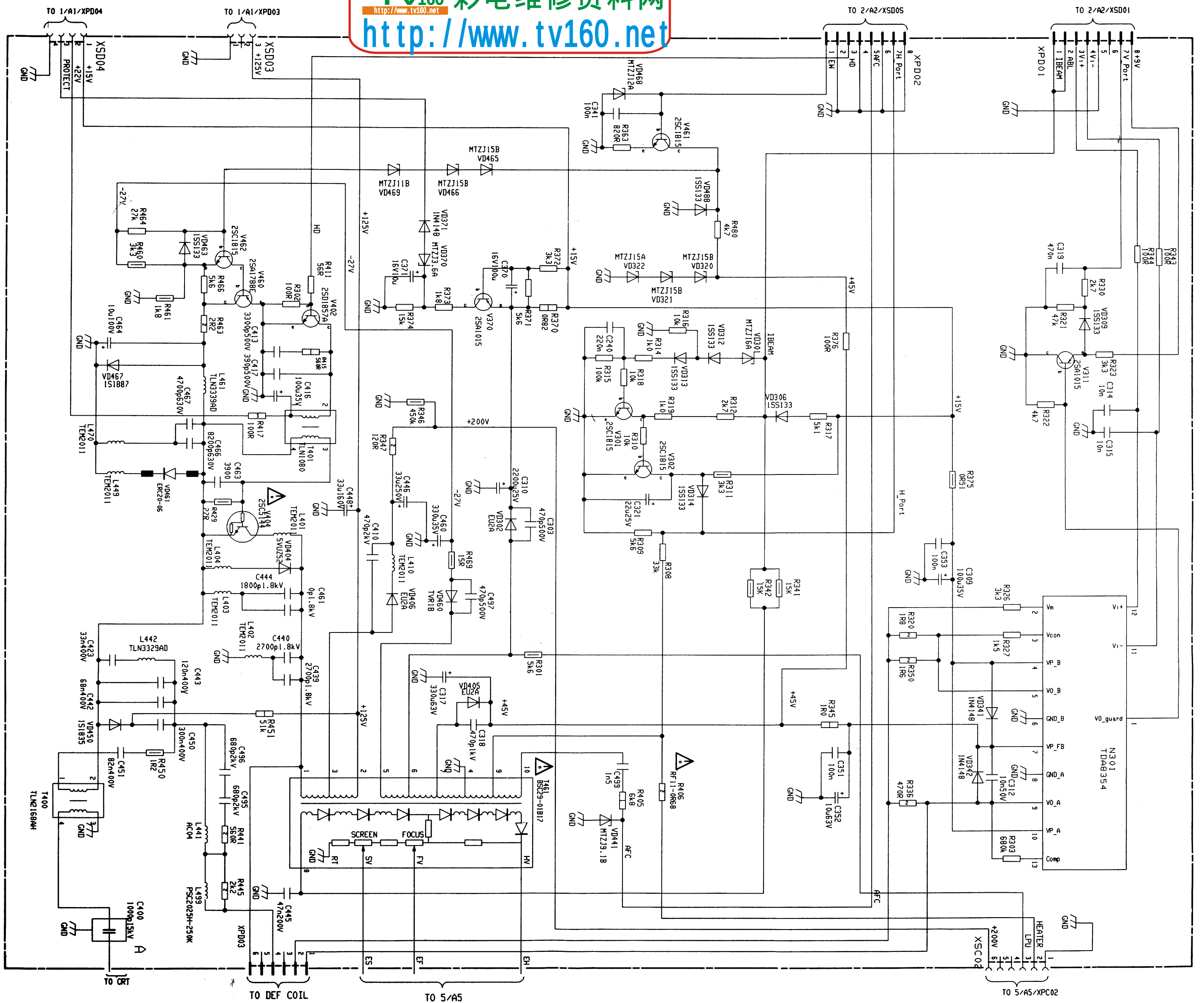
海信牌 TDF2988G型彩色电视机电路图 (A3板) 第3页
