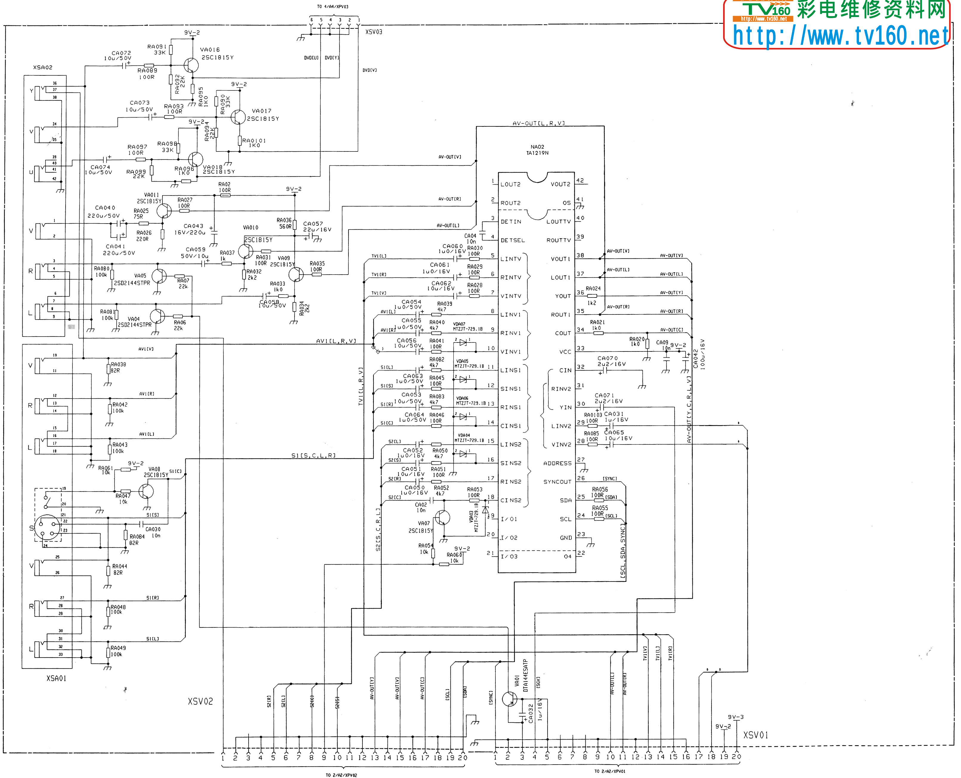
海信牌 TDF2988G型彩色电视机电路图 (A6板) 第6页
