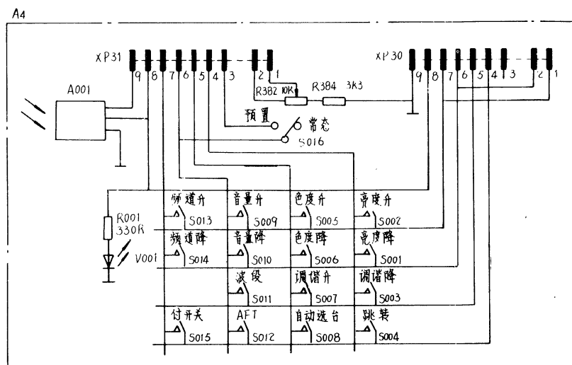
SR5132型彩色电视接收机电路图 (遥控线路)
