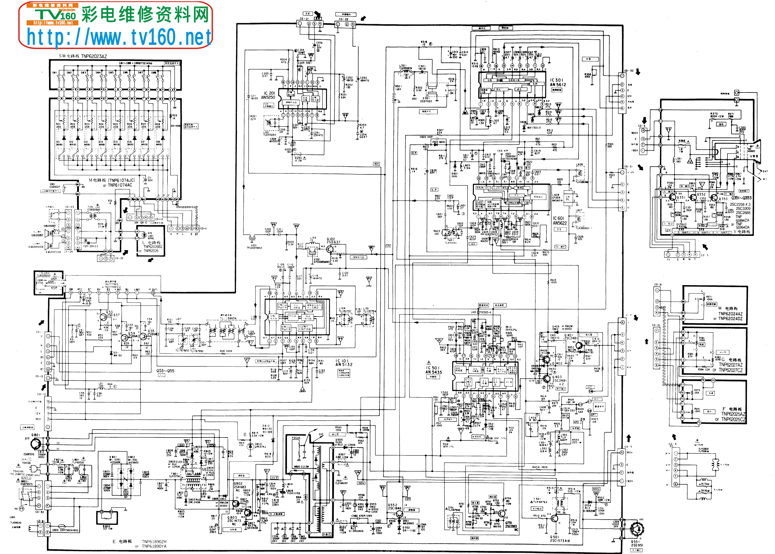
TC-218系电路图(机芯号码M11)
