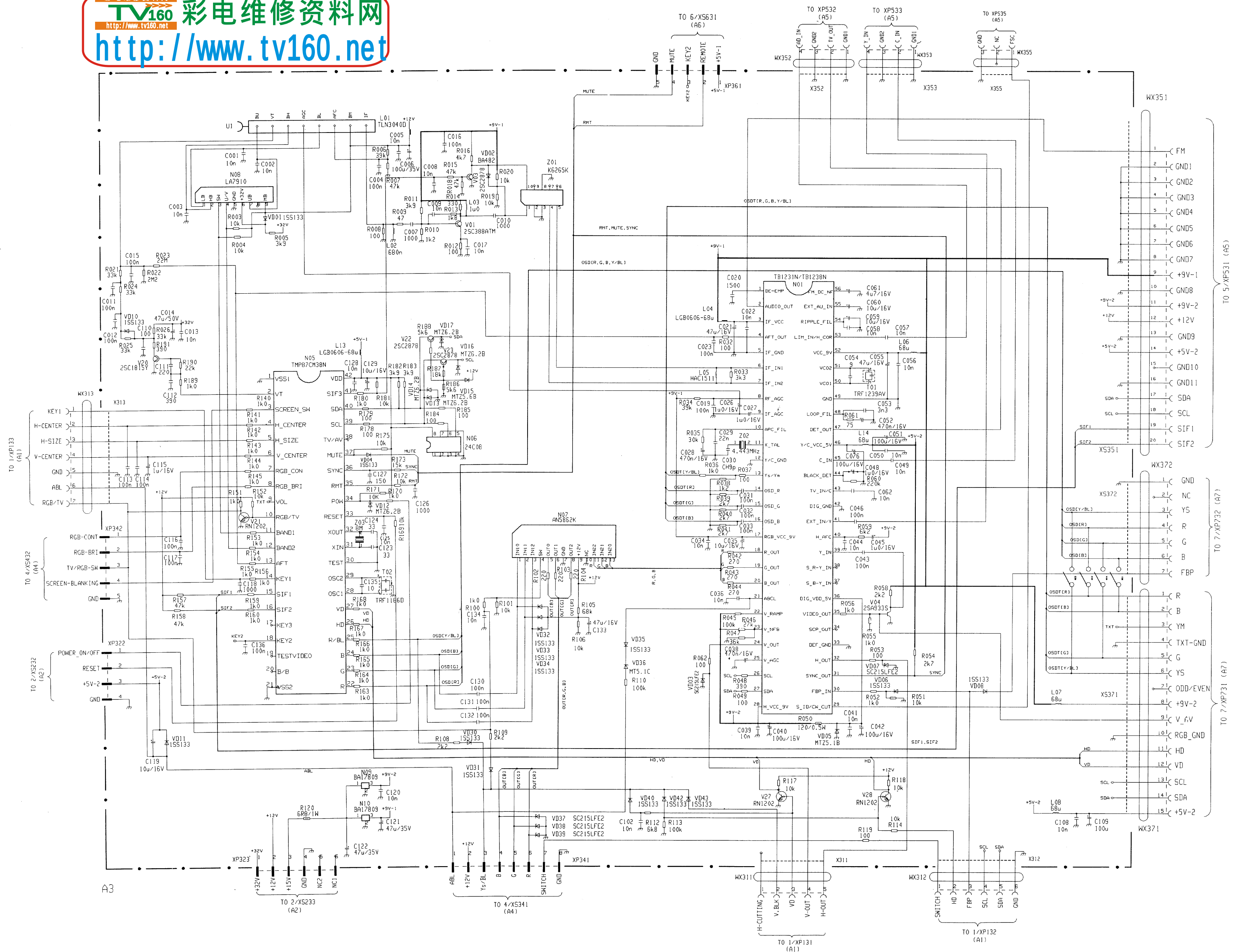
海信牌 TDF2966 型彩色电视机电路图 (A3 板)
