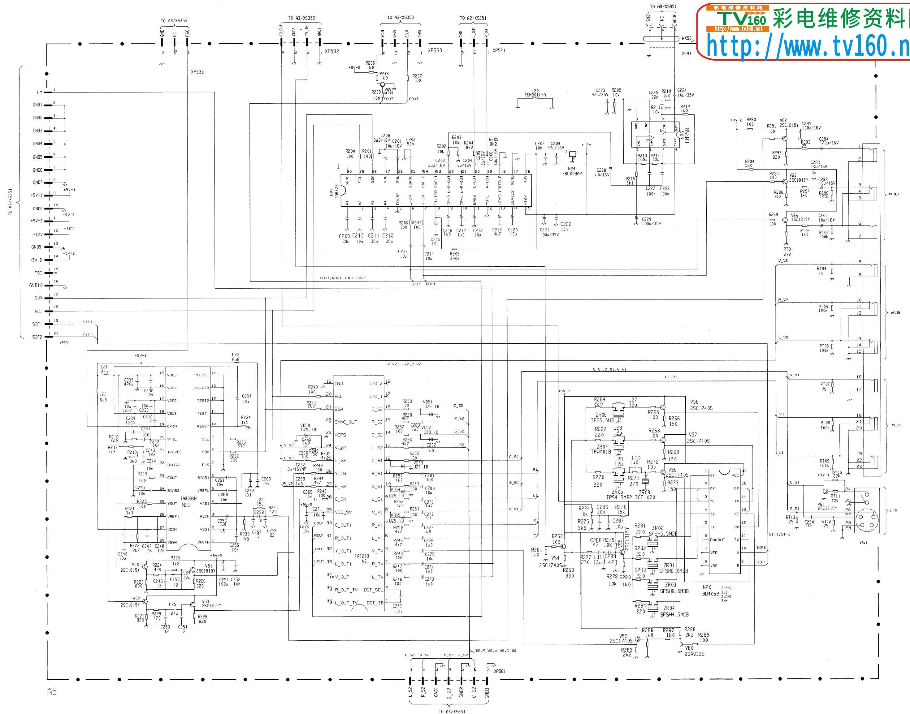
海信牌 TDF2966 型彩色电视机电路图 (A5 板)
