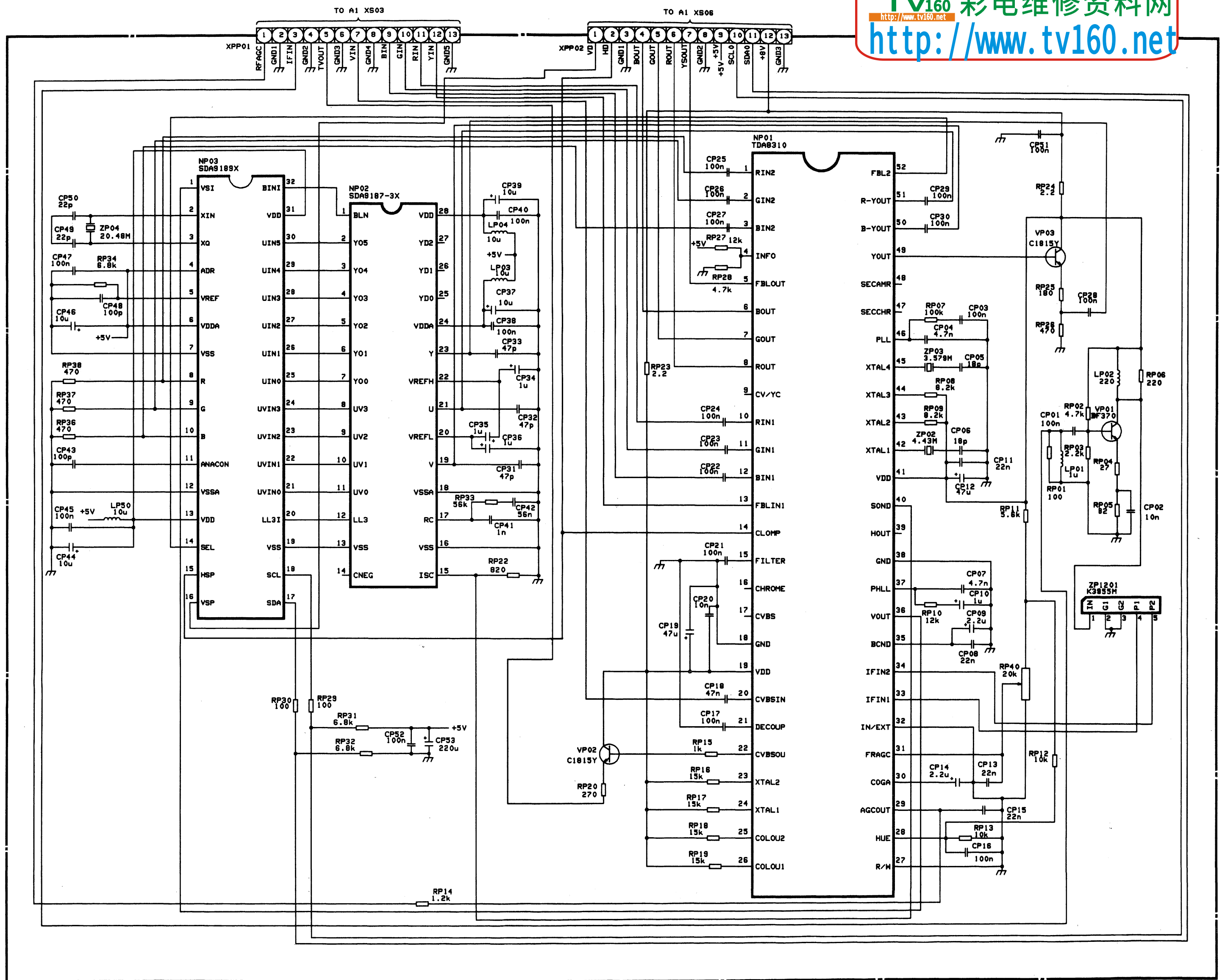
海信牌 TF3430DP 型彩色电视机电路图 (4/4)
