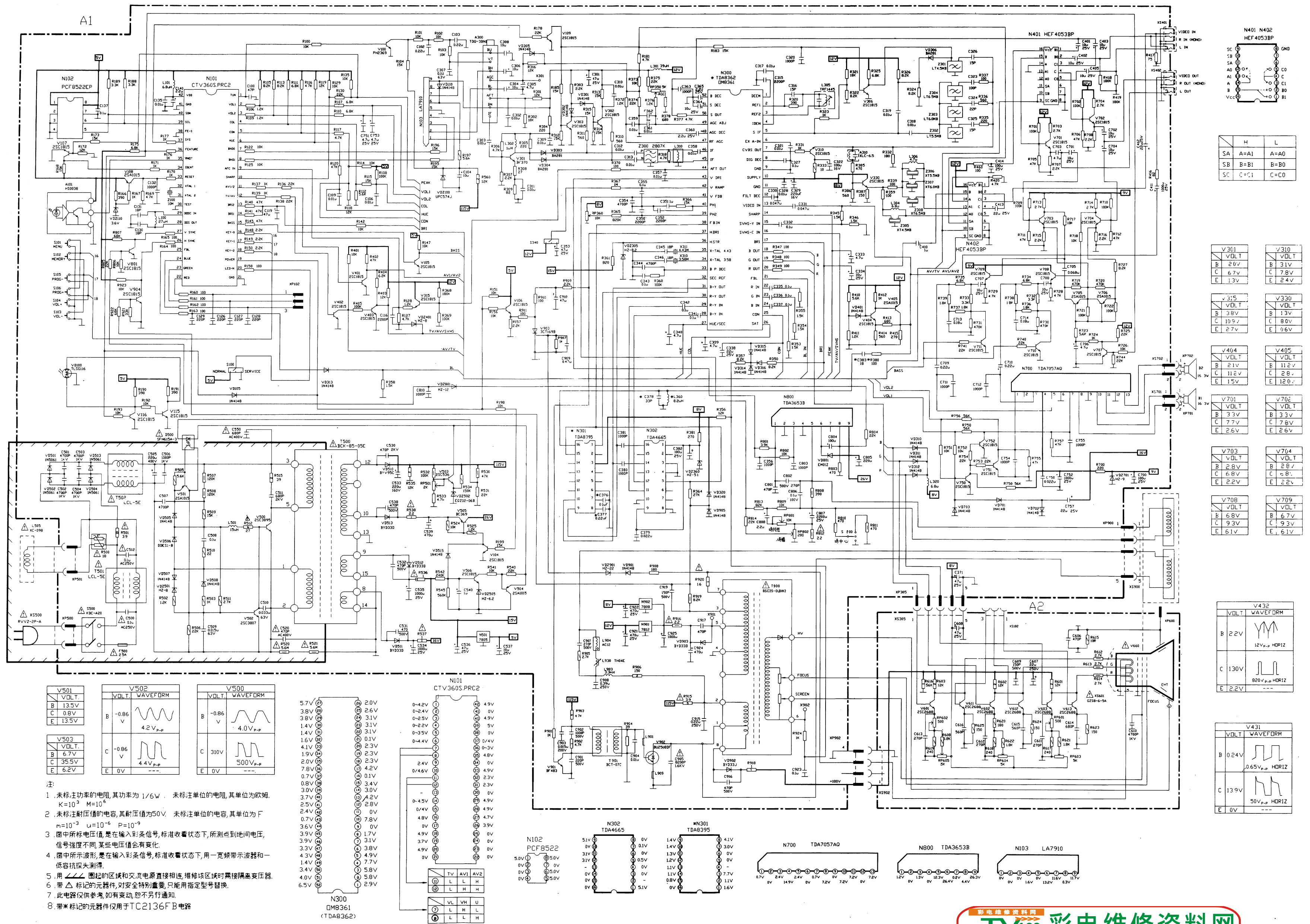
TC2156/TC2157 型彩色电视机电路图
