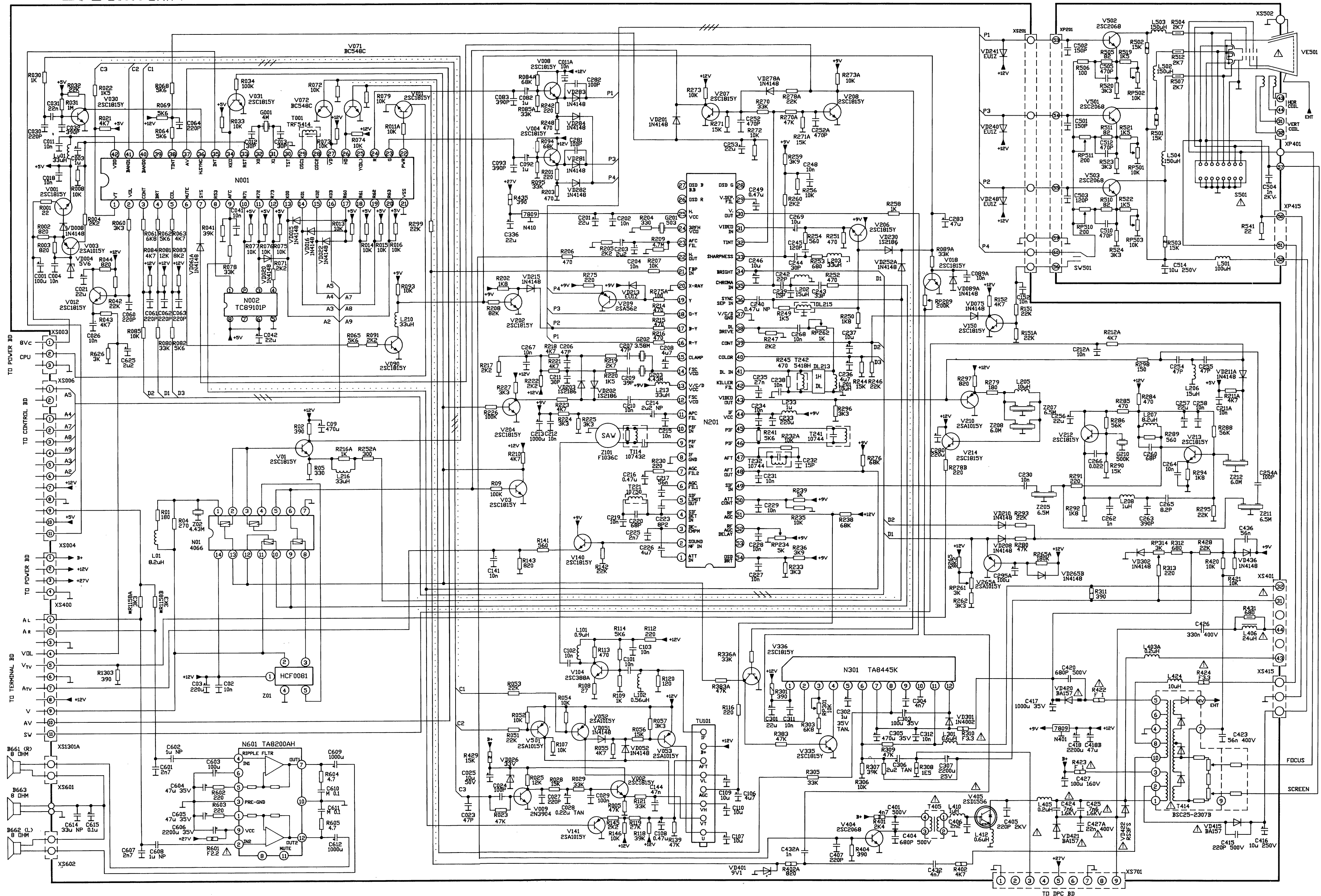
TC2907 型彩色电视机电路图
