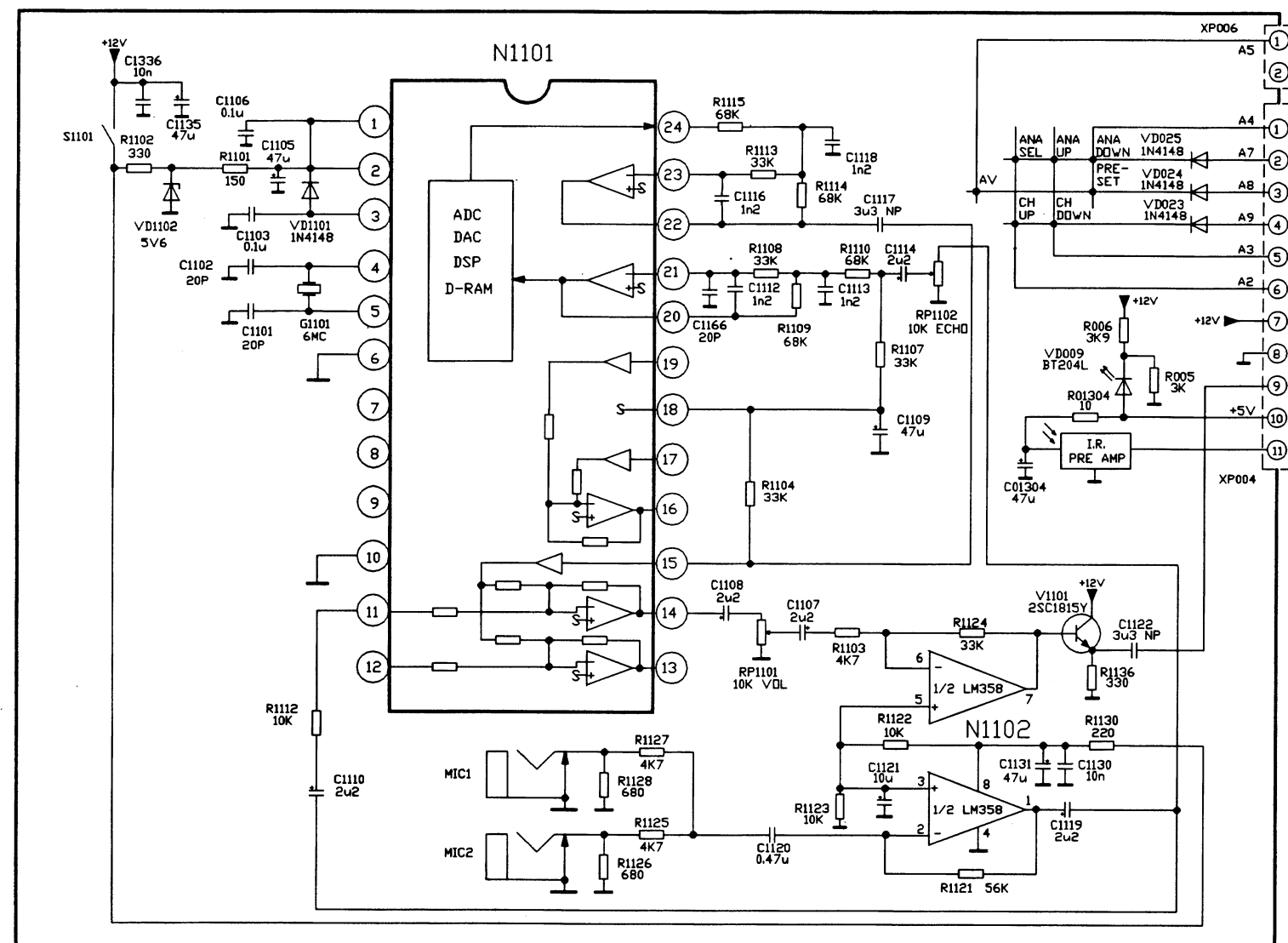
控制及卡拉 OK 电路图
