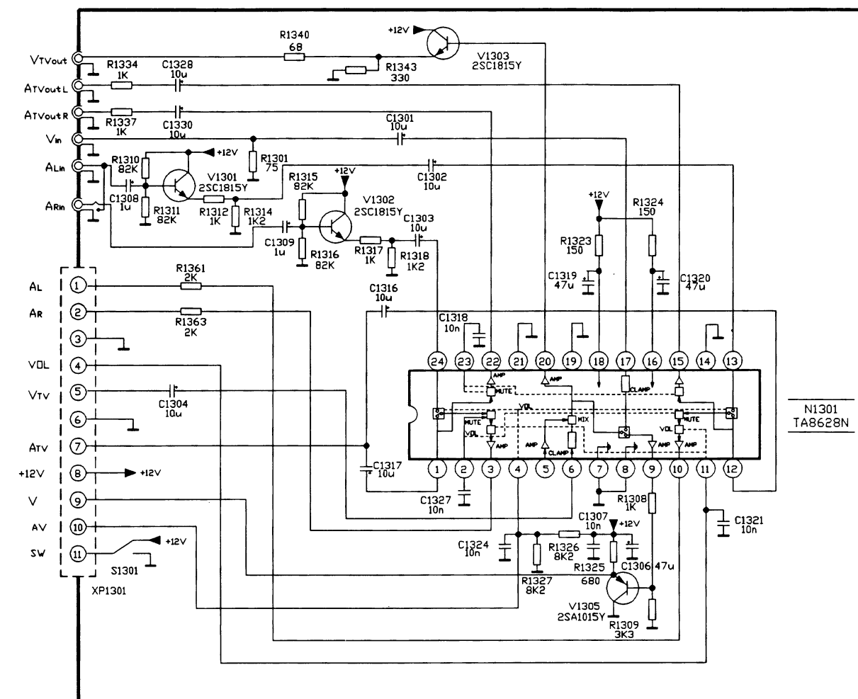
端子板电路图
