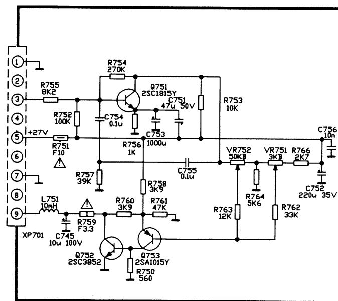
枕校电路图
