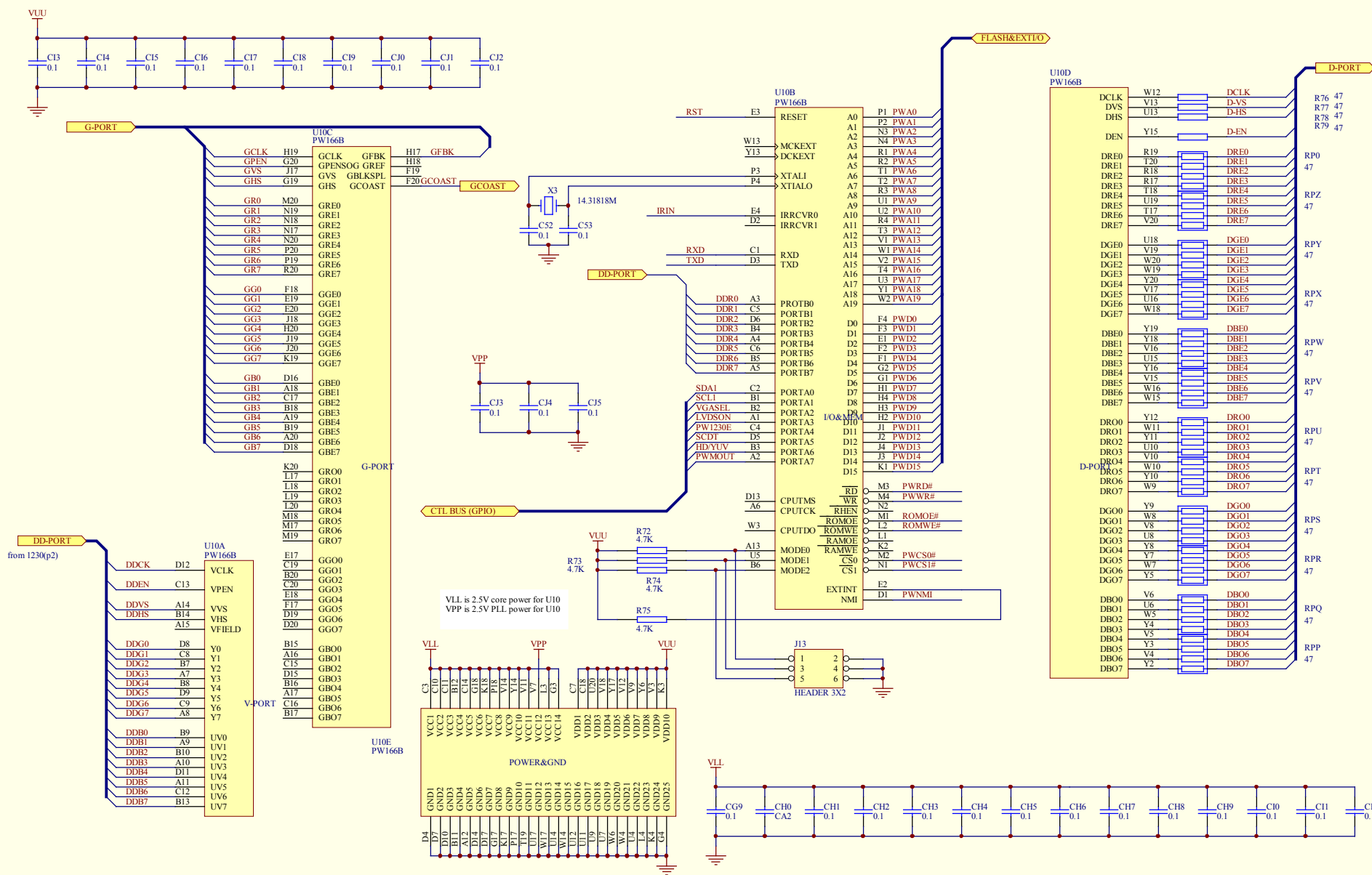
海信牌TPW4211等离子电视机电路原理图(7)
