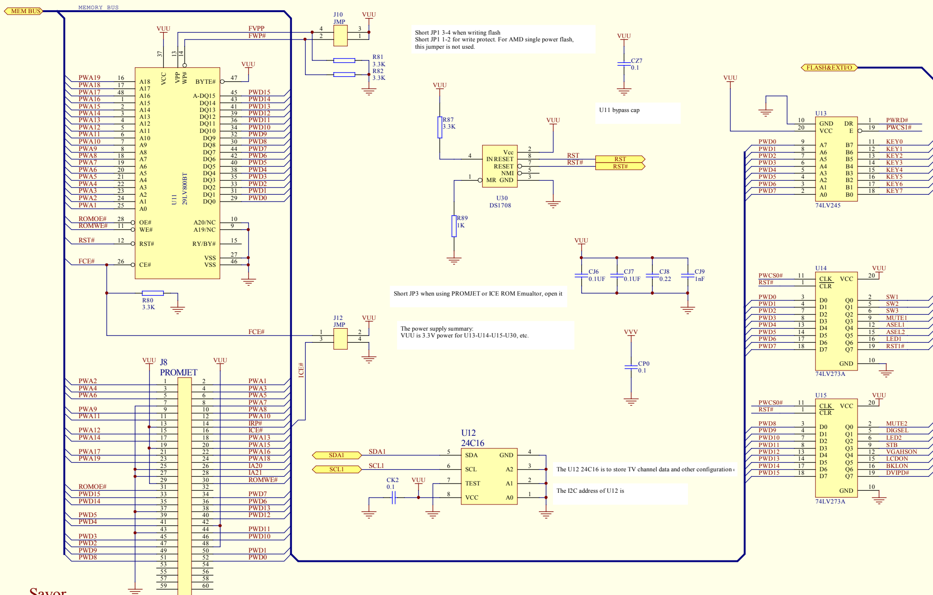
海信牌TPW4211等离子电视机电路原理图(8)
