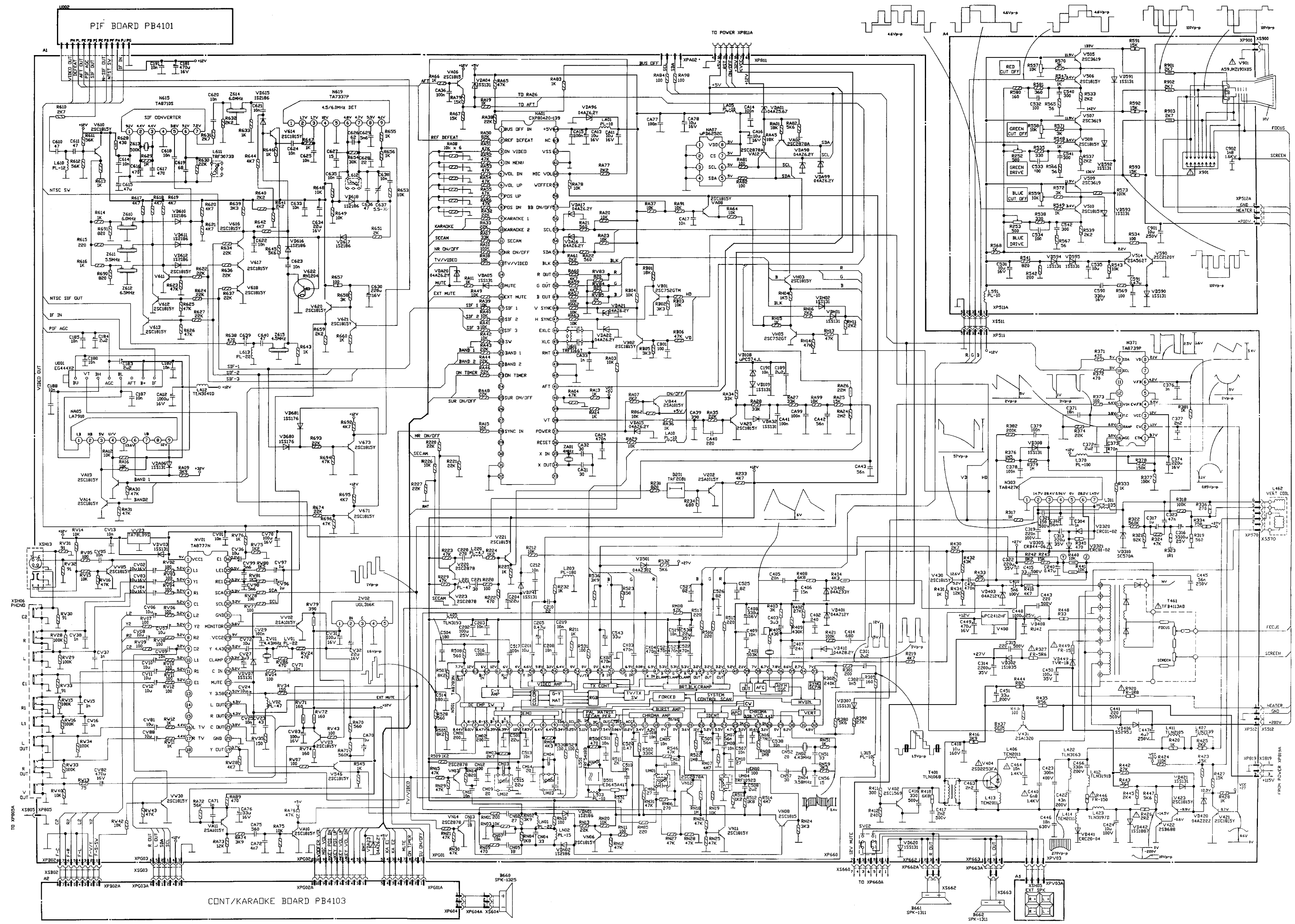
TC2518 KB 型彩色电视接收机电路图
