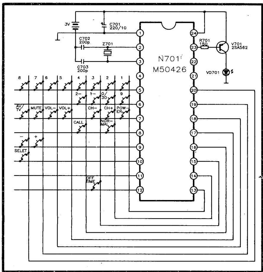
遥控器原理图
