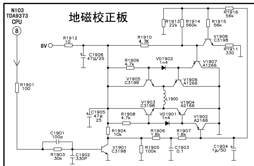
34英寸、29英寸纯平彩管SK型机可设地磁校正板
