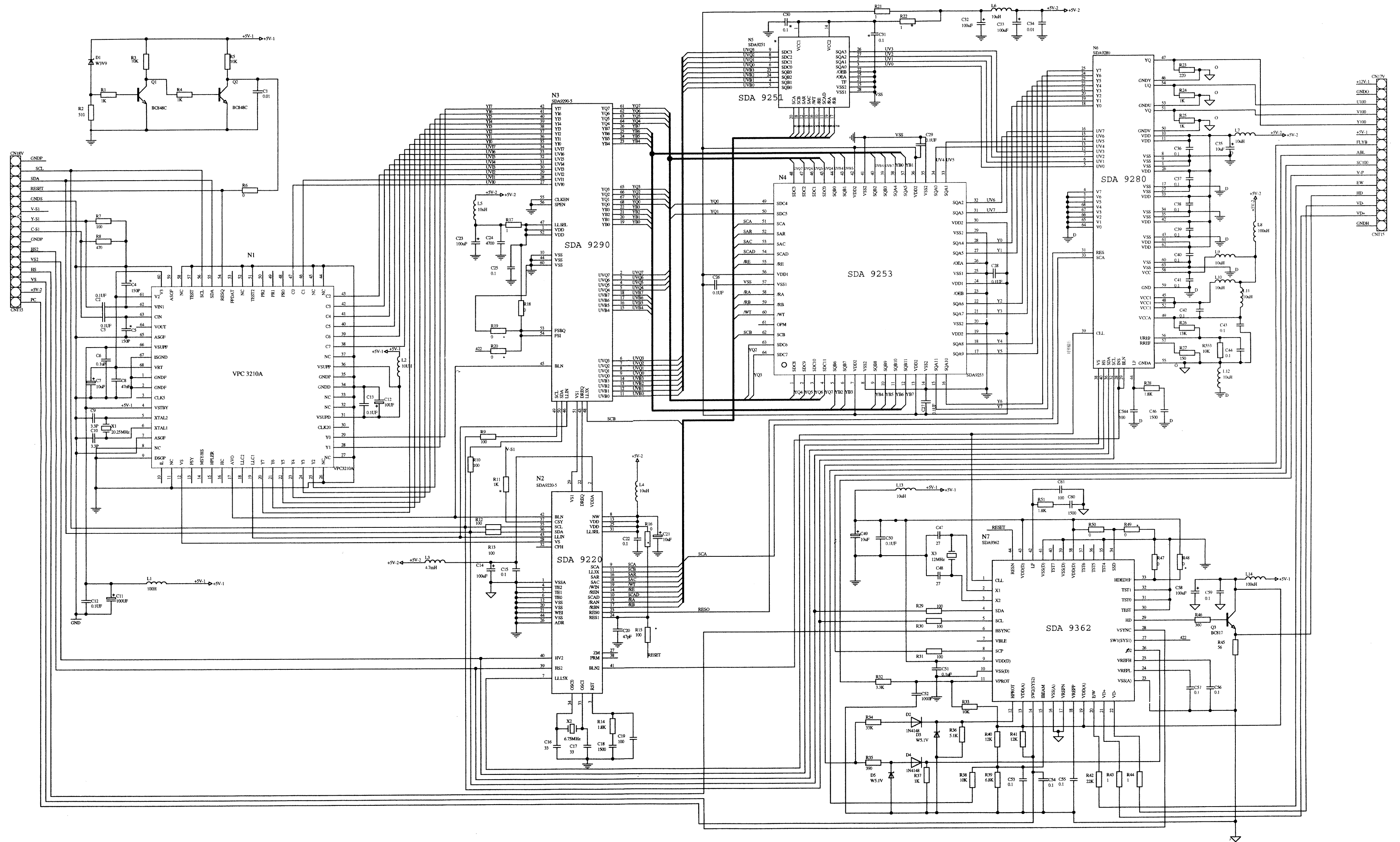
5M01电原理图：数字处理单元
