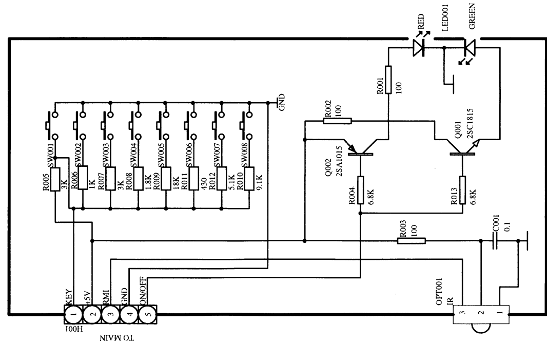
5M10机芯：键控板图
