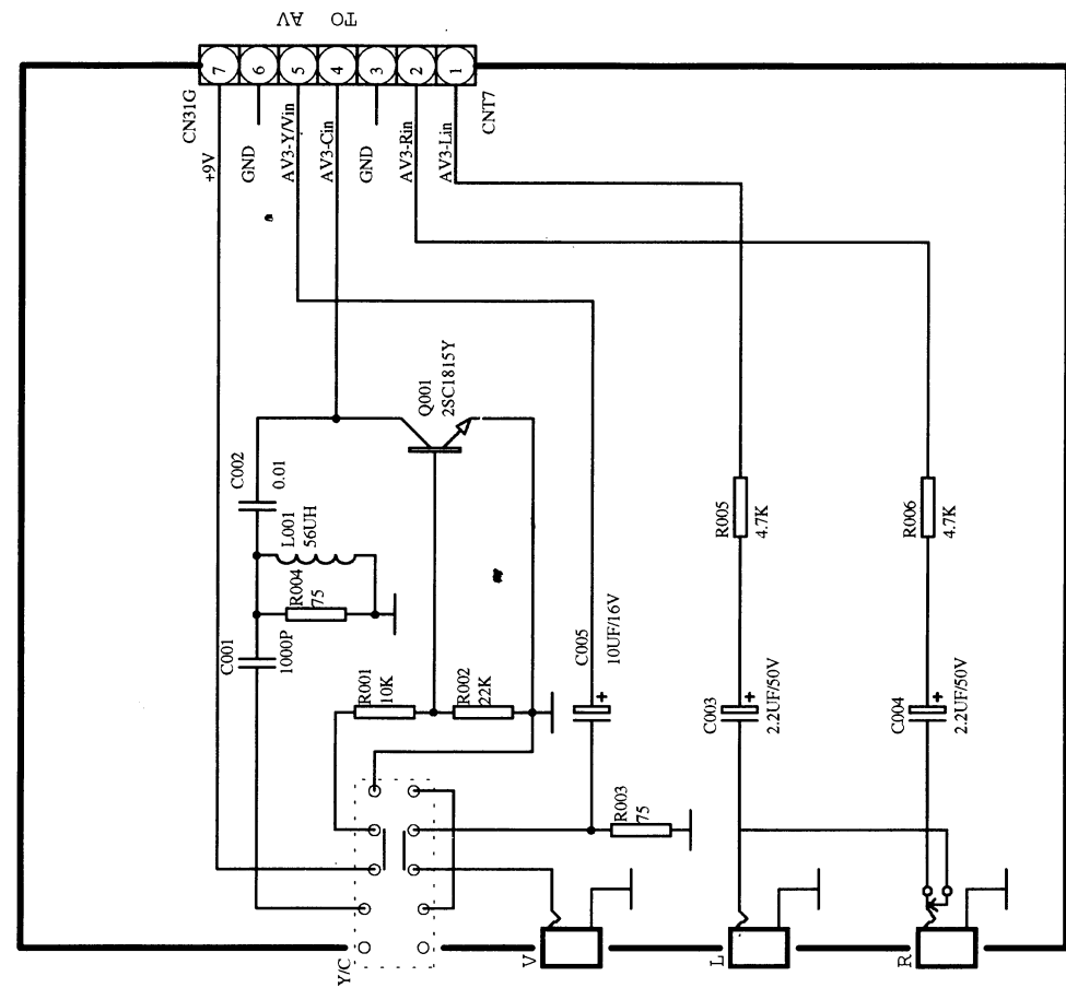
5M10机芯：前AV板图
