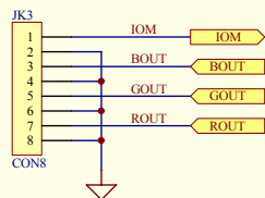
TO_TDA9332
