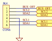
TO_MCU
