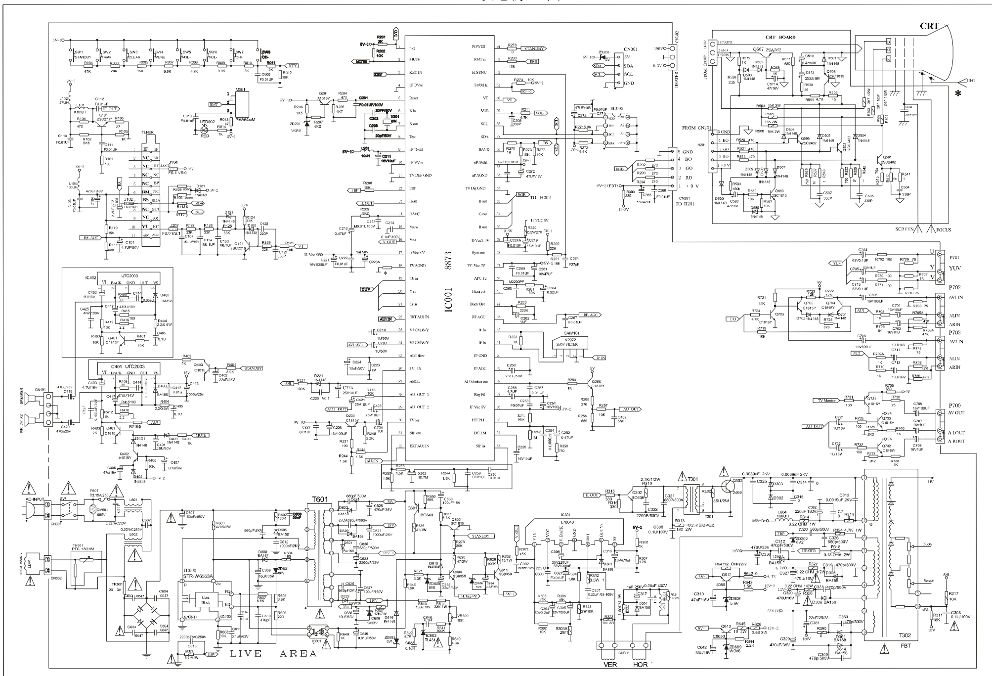
3T60机芯原理图
