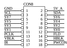
HEADER 9X2
