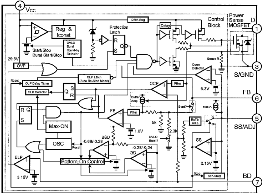
STR-W6553 内部框图
