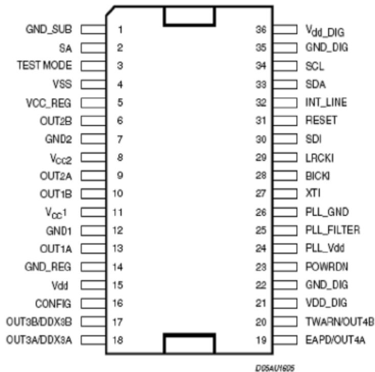
图 9 STA335BW 引脚图
