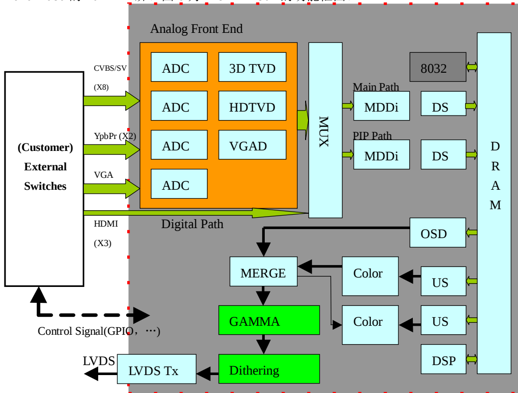
图 4 MT8222AHSU-B 功能框图
